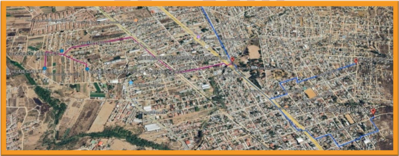
Líneas de conducción a tanques de almacenamiento Líneas de conducción de pozos profundos Pozos profundos Tanques de distribución
