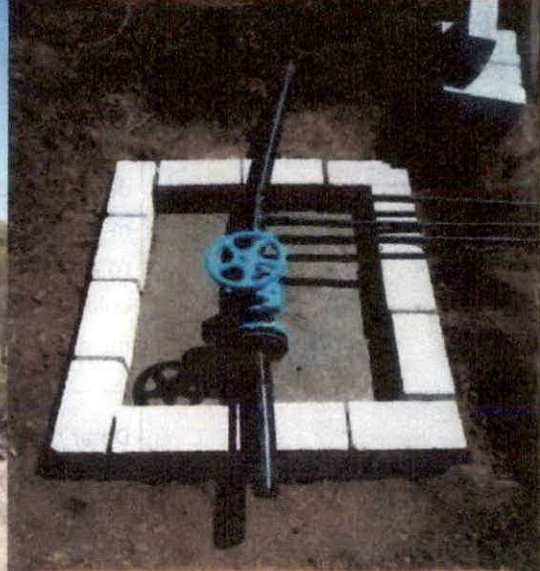
Instalación de tomas y válvulas
