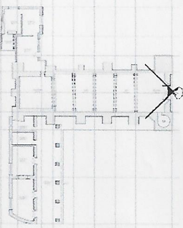
PLANTA ARQUITECTÓNICA
