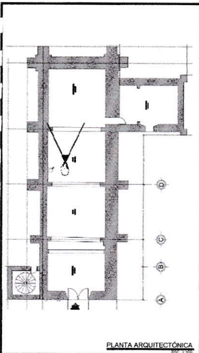
PLANTA ARQUITECTÓNICA REC. 1300
