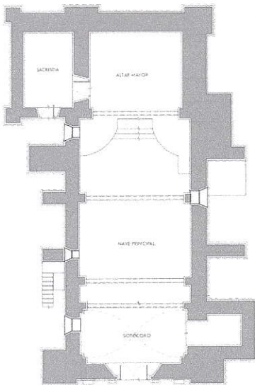
PLANTA ARQUITECTÓNICA
