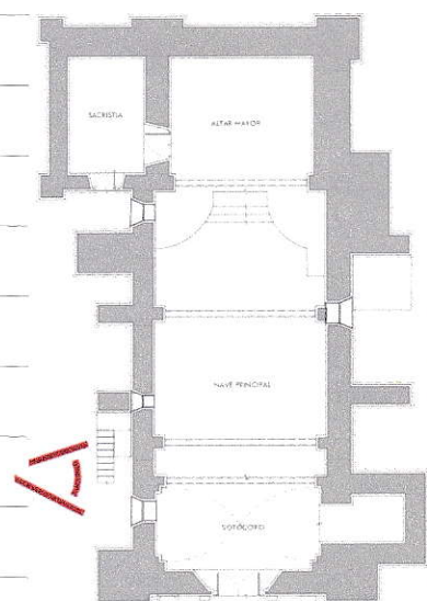
PLANTA ARQUITECTÓNICA 1:100 - 1:100
