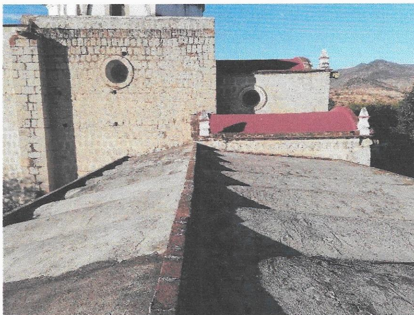
Imagen 05: Fotografía de vista de bóveda catalana en área más antigua de casa cural.
