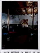
F-02. VISTA INTERIOR EN ANEXO. SE OBSERVA APUNTALAMIENTO PROVISIONAL EN CUBIERTA CON PRESENCIA DE DAÑOS A CAUSA DE SISMO.
