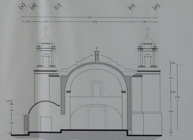
SECCIÓN B-B
