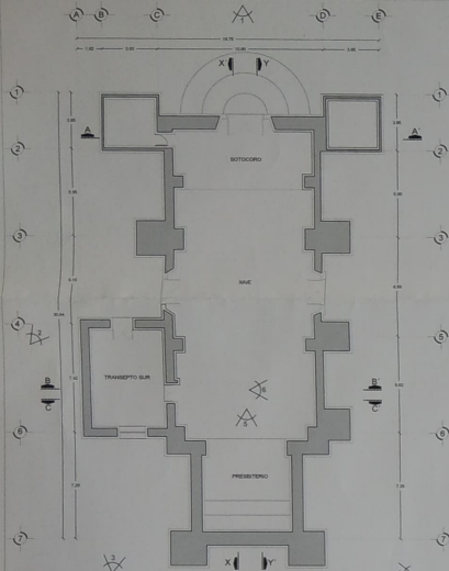
PLANTA ARQUITECTÓNICA
