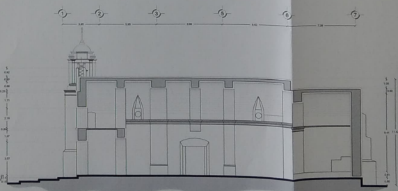
SECCIÓN Y-Y
