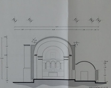
SECCIÓN C-C
