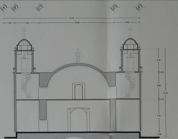
SECCIÓN A-A
