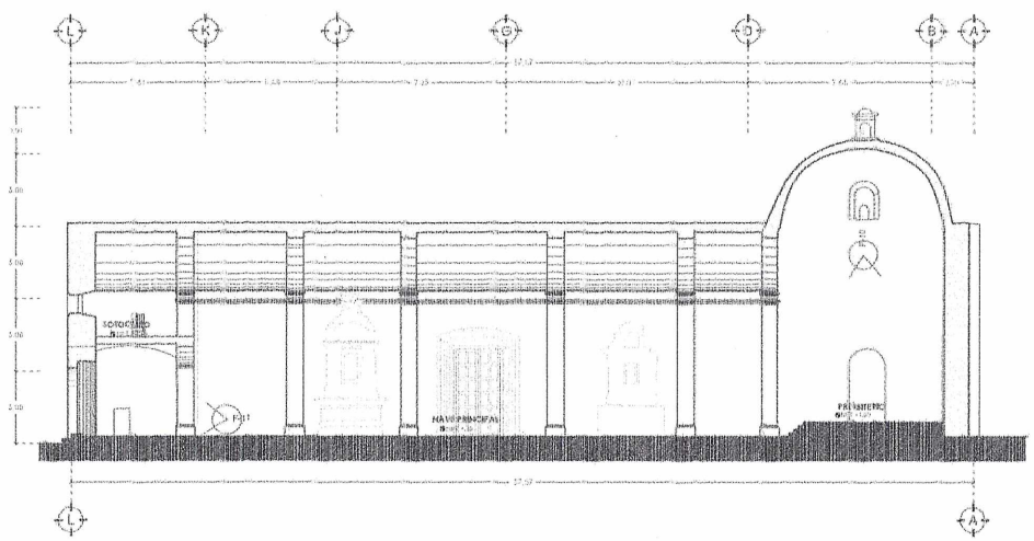
CORTE TRANSVERSAL B-D ESTADO ACTUAL
