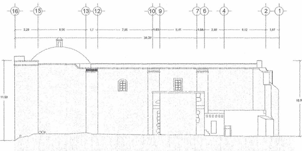
ALZADO SUR ESTADO ACTUAL
