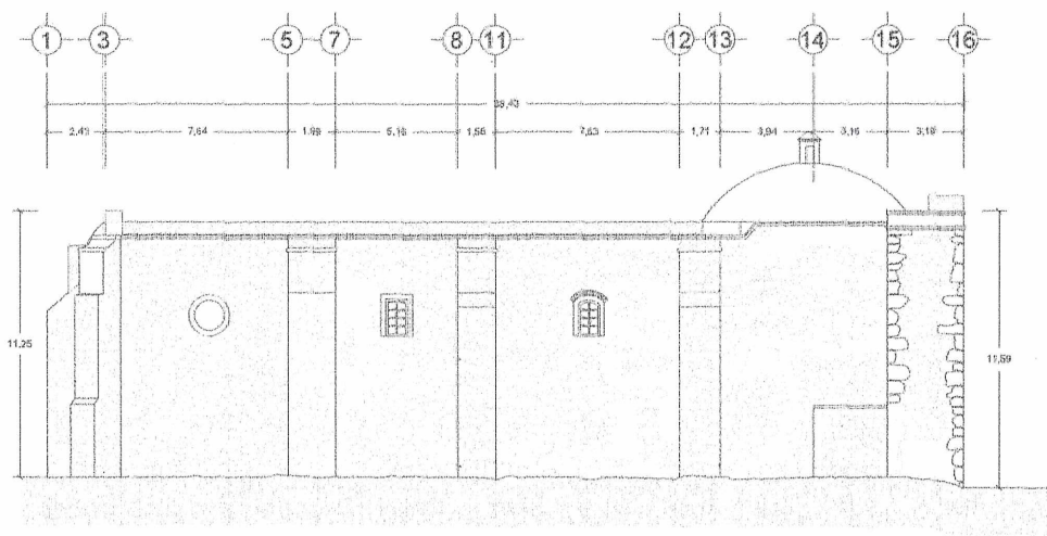
ALZADO NORTE ESTADO ACTUAL
