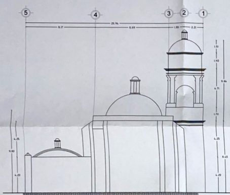
ALZADO PONIENTE ESCALA 1:100
