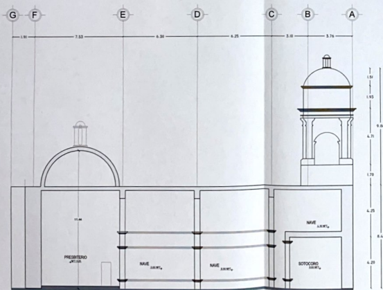
CORTE A-A' ESCALA 1:100
