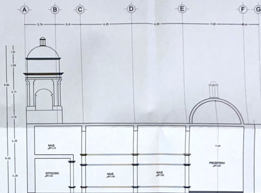
CORTE B-B' ESCALA 1:100
