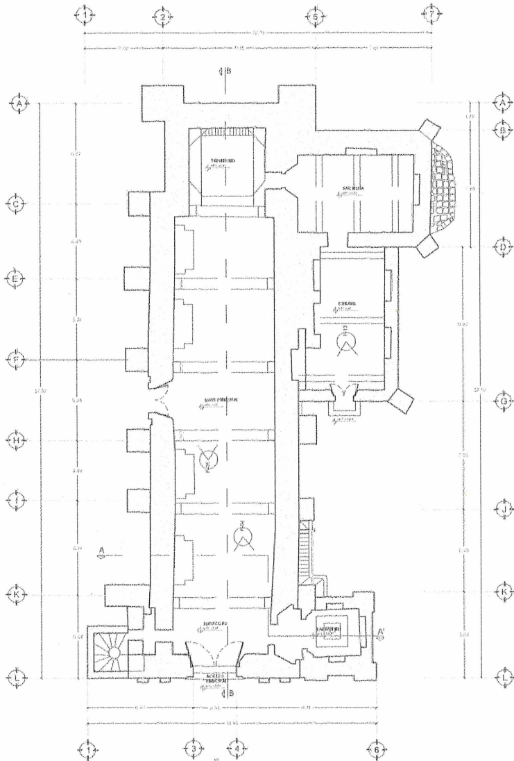
PLANTA ARQUITECTÓNICA ESTADO ACTUAL
