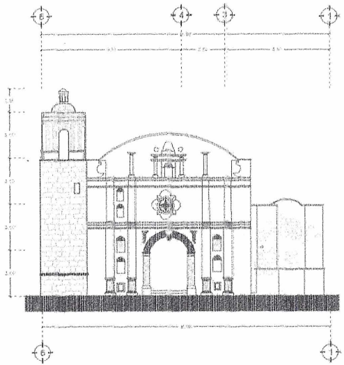
ALZADO PONIENTE ESTADO ACTUAL
