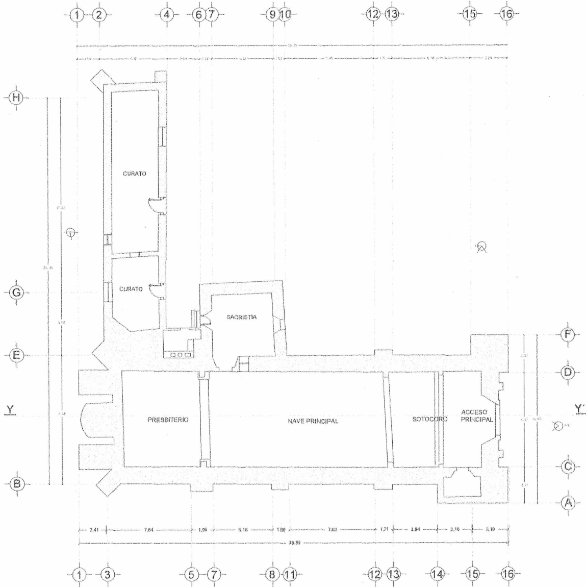
PLANTA ARQUITECTONICA ESTADO ACTUAL
