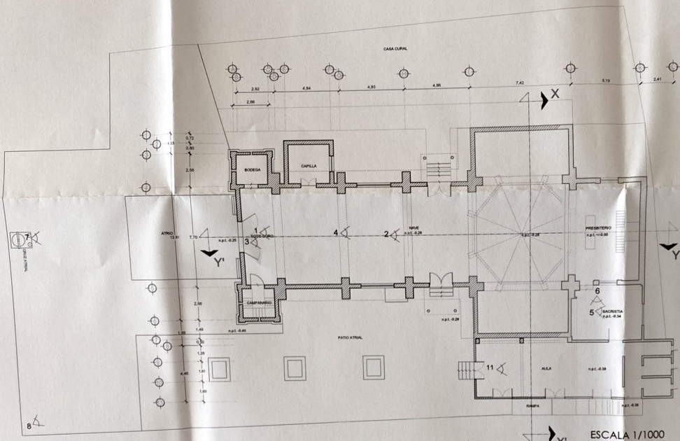
PLANTA ARQUITECTÓNICA
