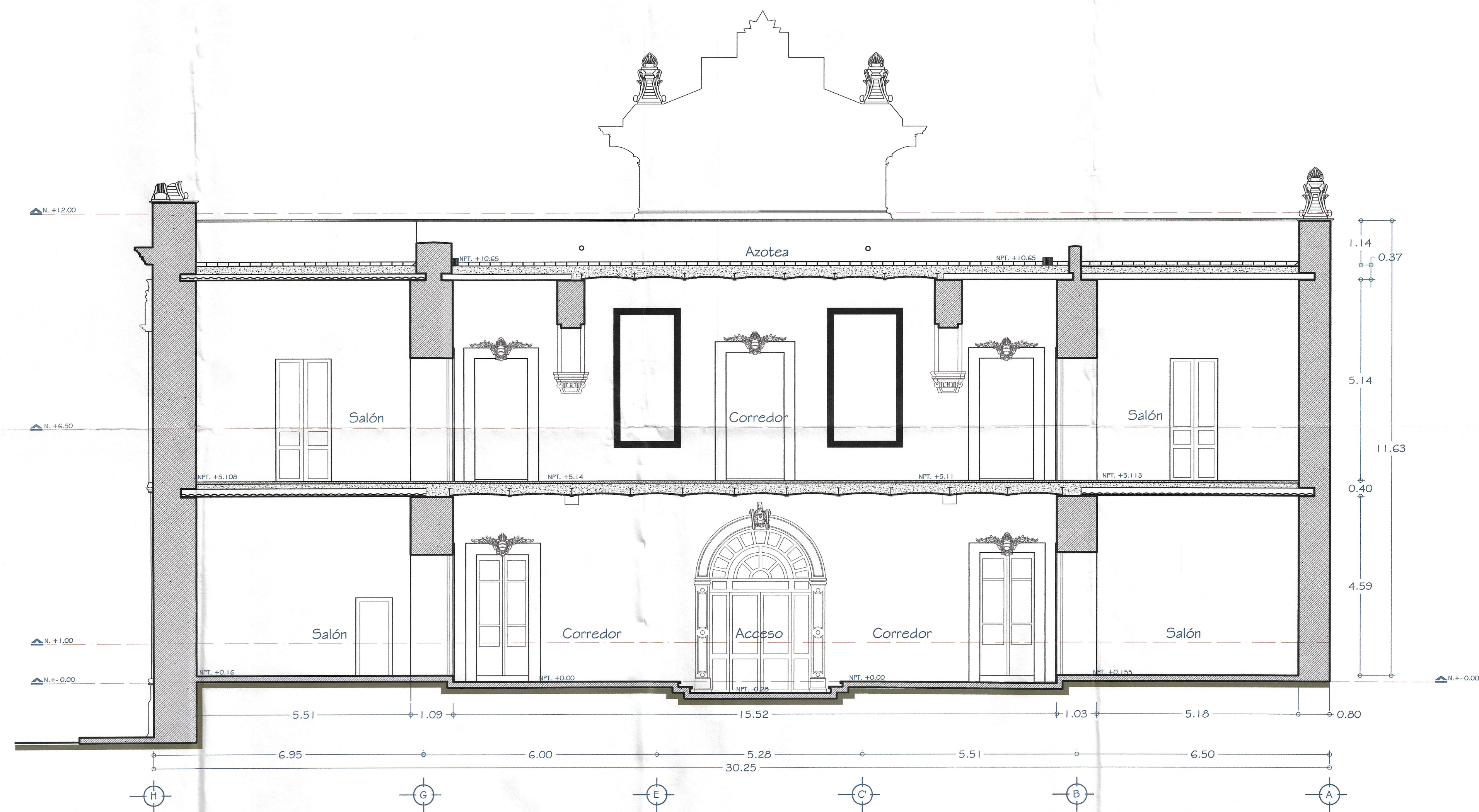
CORTE C-C' (FACHADAS INTERIORES 1er. PATIO)
