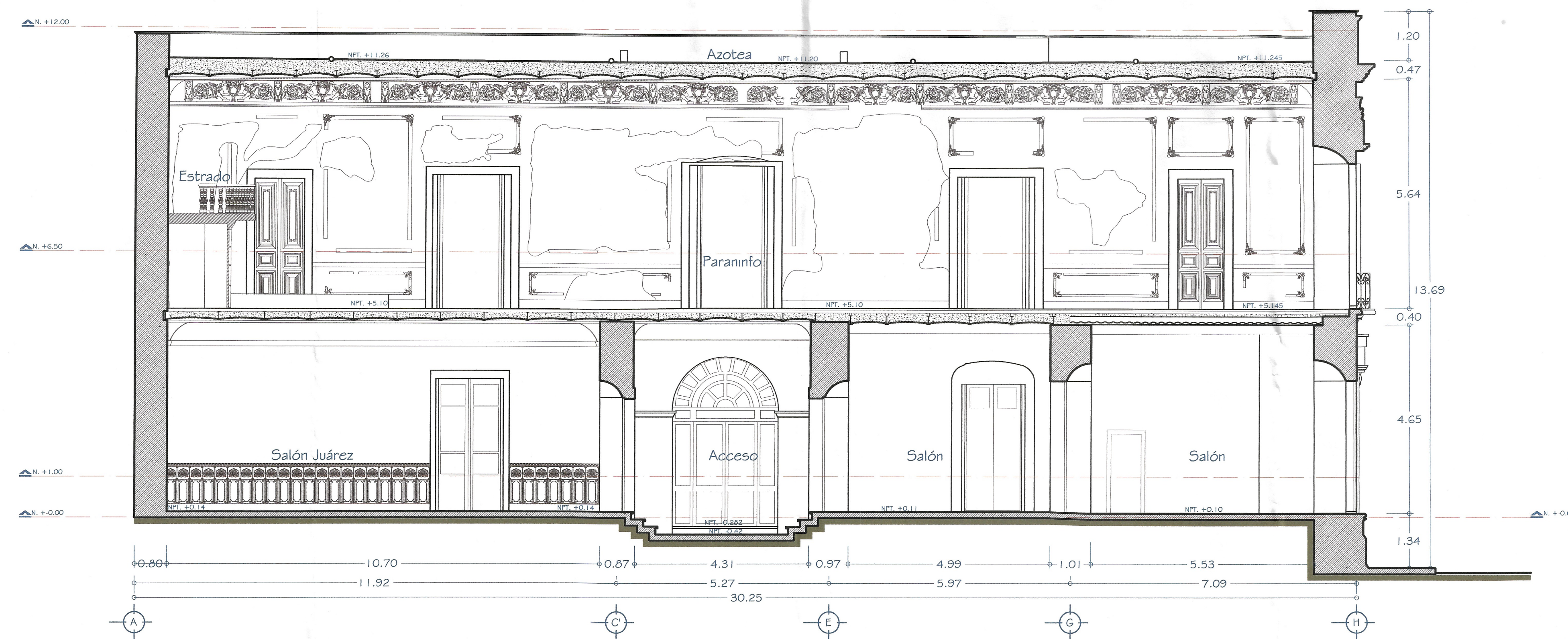
CORTE A-A' (FACHADAS INTERIORES NORTE)
