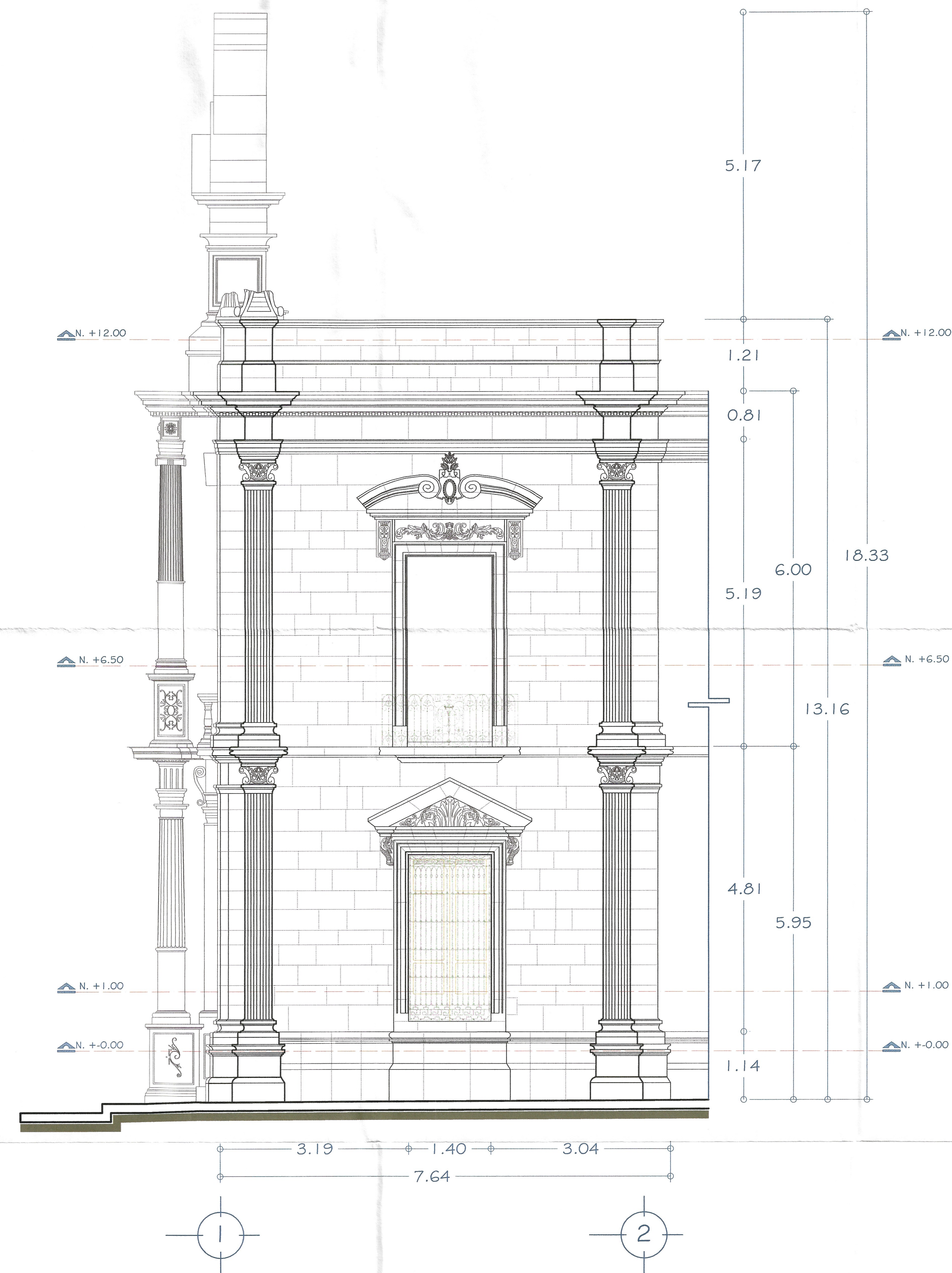
FACHADA LATERAL (MACEDONIO ALCALA)
