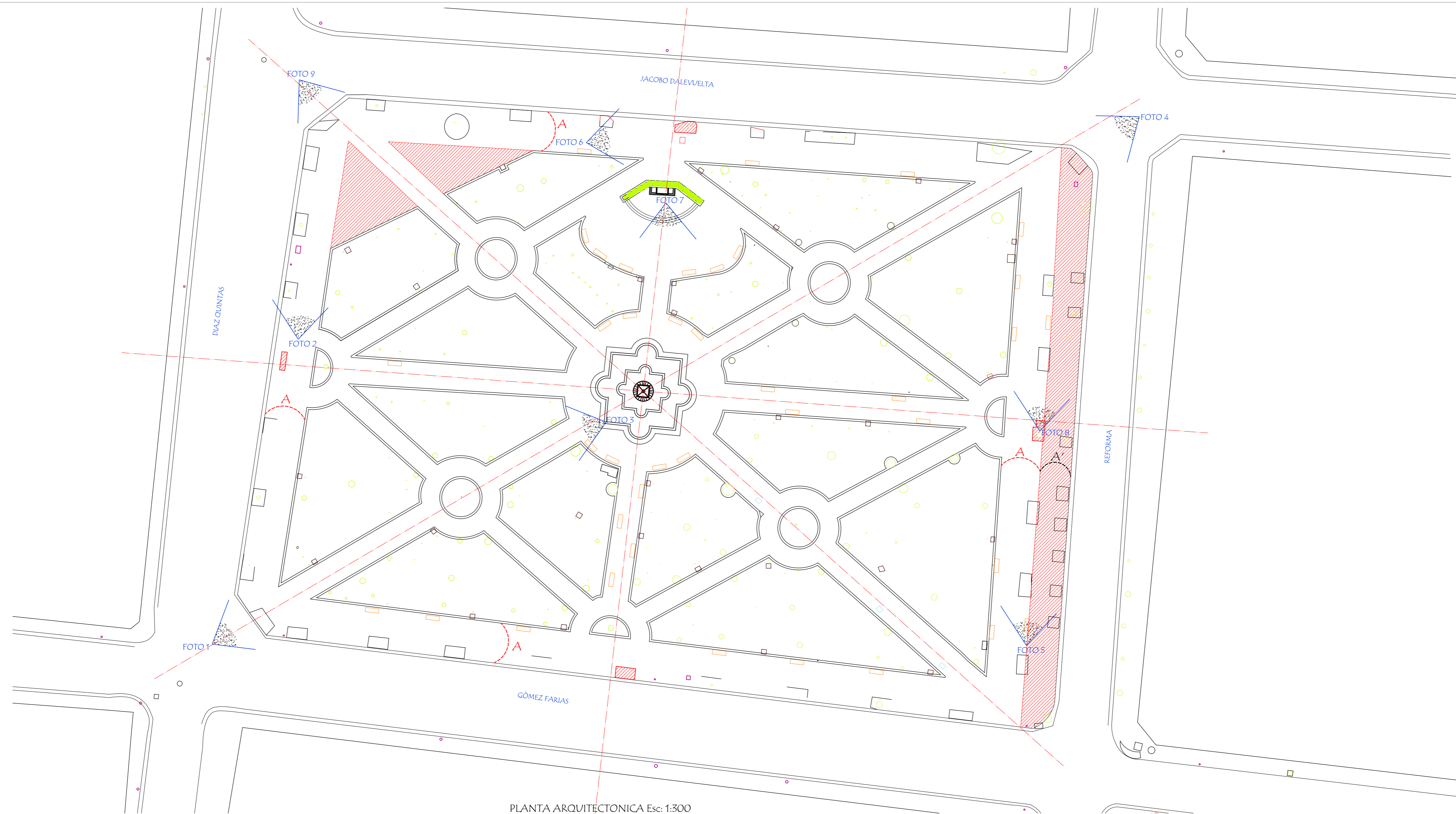
PLANTA ARQUITECTONICA Esc: 1:300
