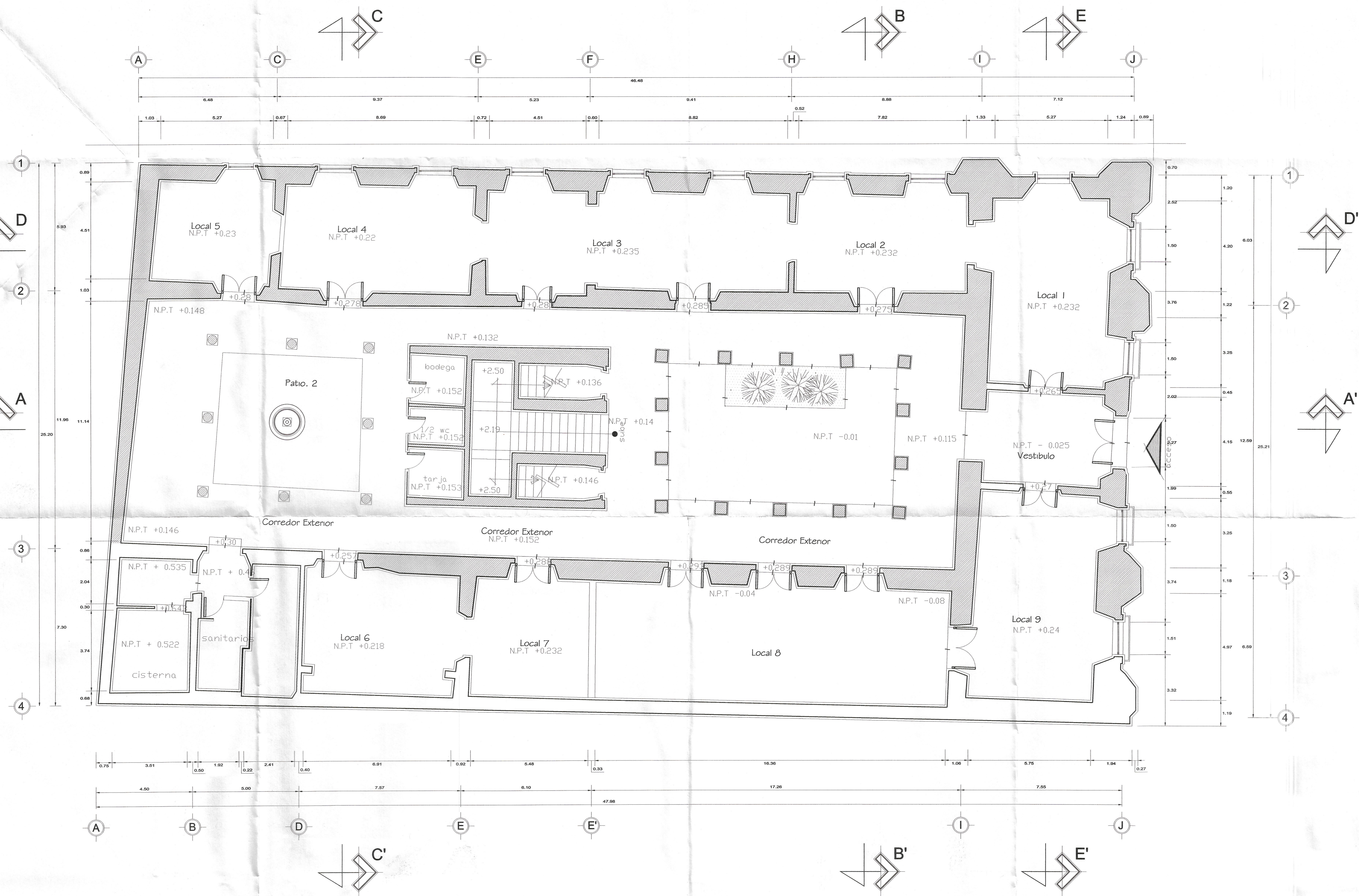
PLANTA ARQUITECTONICA BAJA Esc. 1:100
