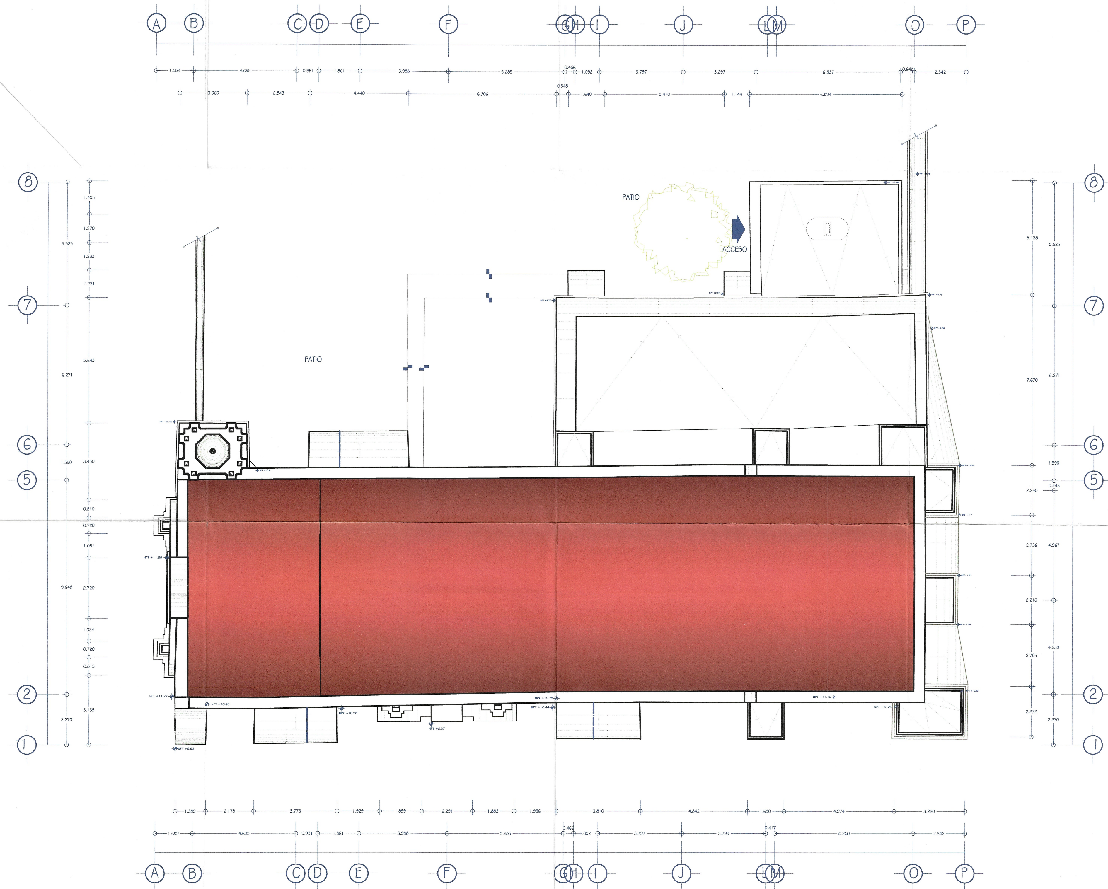
PLANTA AZOTEA ESCALA 1:100
