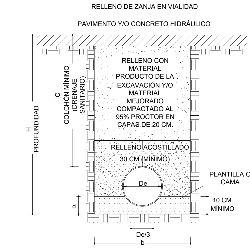
ZANJA TIPO
