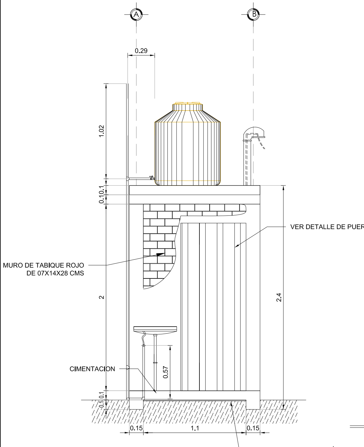
VISTA FRONTAL CASETA ESCALA 1:25
