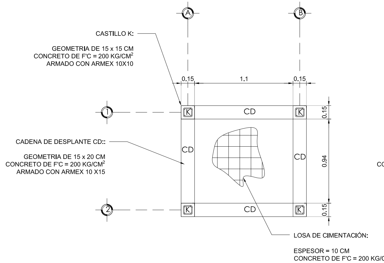
PLANTA DE LOSA DE CIMENTACIÓN CASETA ESCALA 1:25
