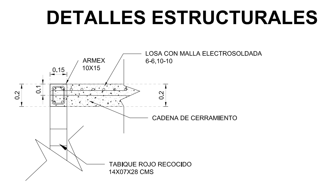
DETALLE DE LOSA DE AZOTEA CASETA ESCALA 1:20
