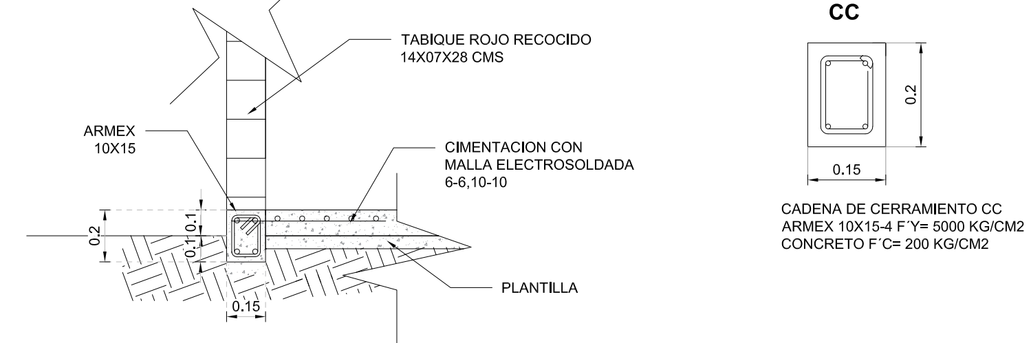
DETALLE DE LOSA DE CIMENTACIÓN CASETA ESCALA 1:20
