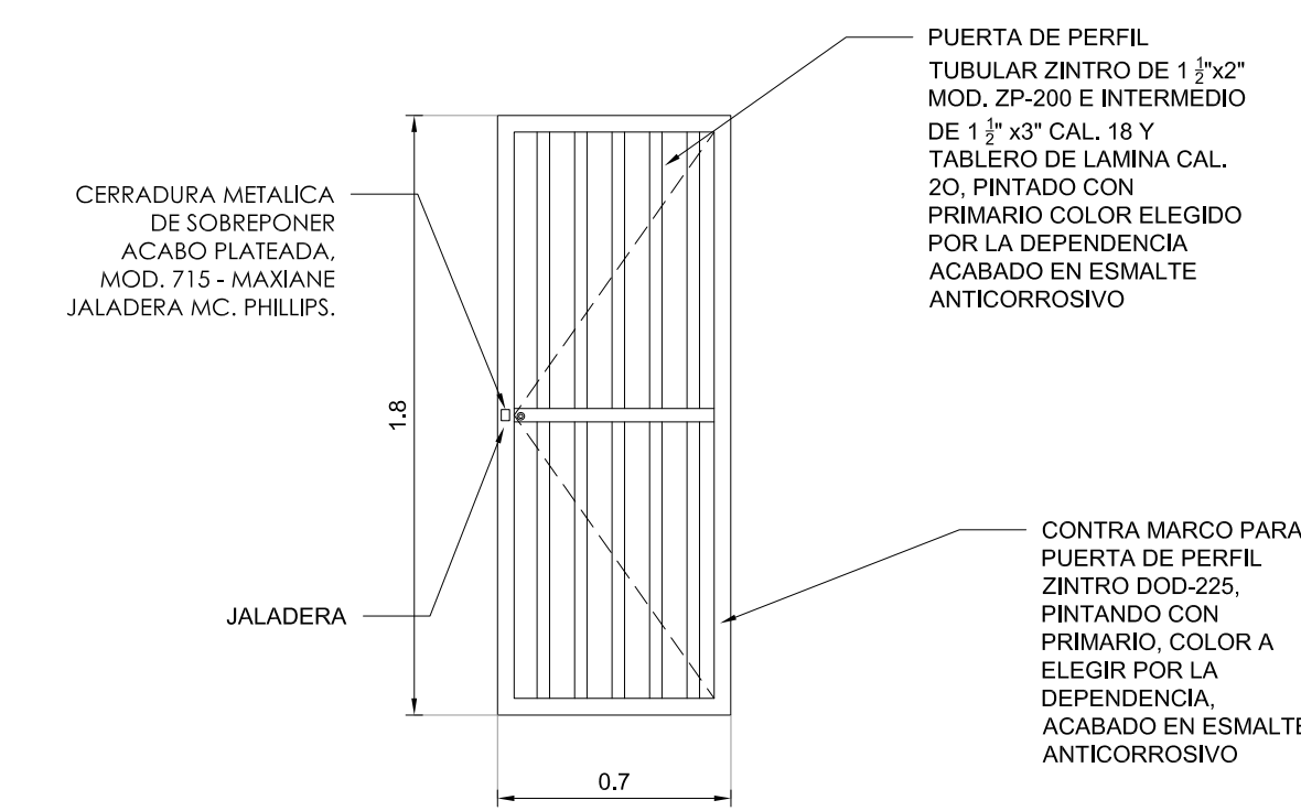
DETALLE DE PUERTA CASETA ESCALA 1:25
