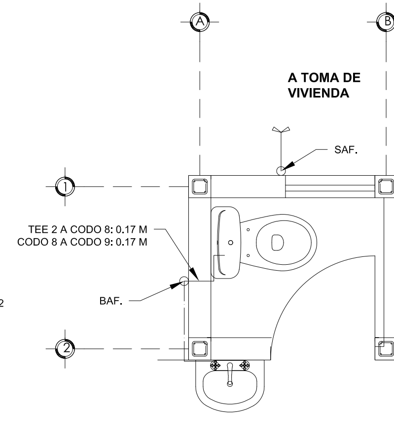
PLANTA INSTALACIÓN HIDRUALICA CASETA ESCALA 1:25
