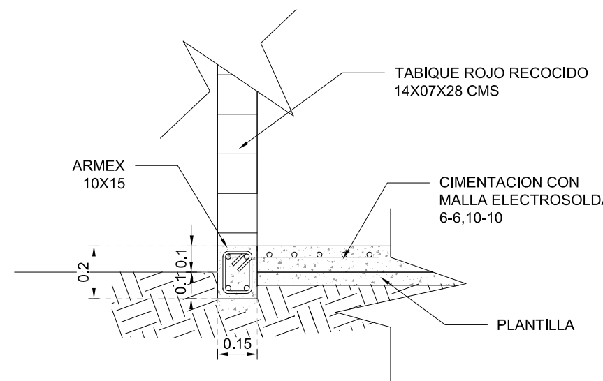
DETALLE DE LOSA DE CIMENTACIÓN CASETA ESCALA 1:20
