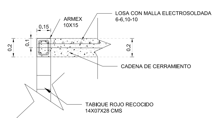
DETALLE DE LOSA DE AZOTEA CASETA ESCALA 1:20
