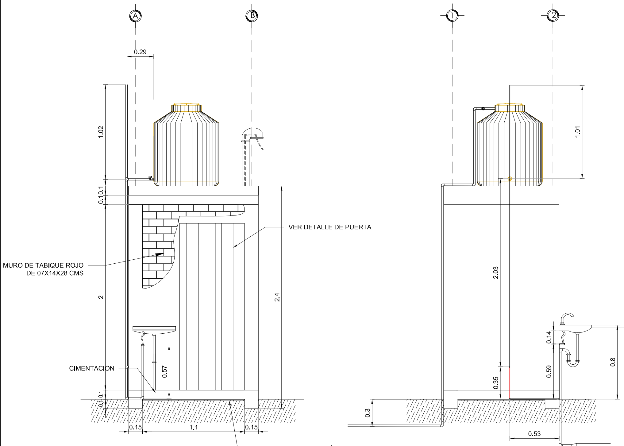
VISTA FRONTAL CASETA ESCALA 1:25
