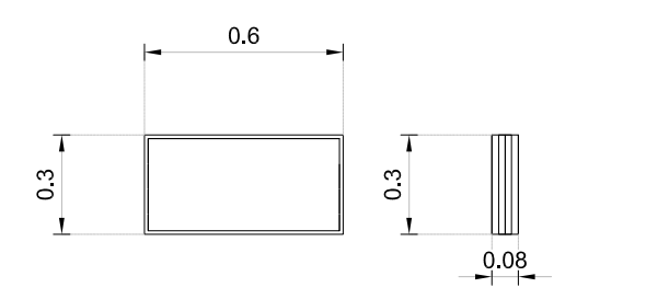
DETALLE DE VENTANA ESTRUCTURAL CASETA ESCALA 1:25
