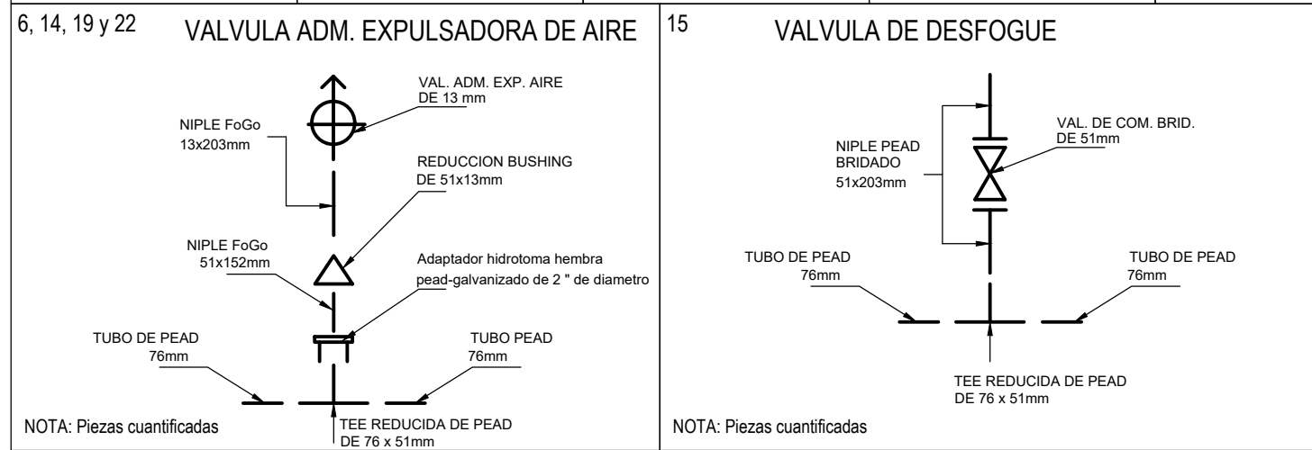
DETALLES PEAD
