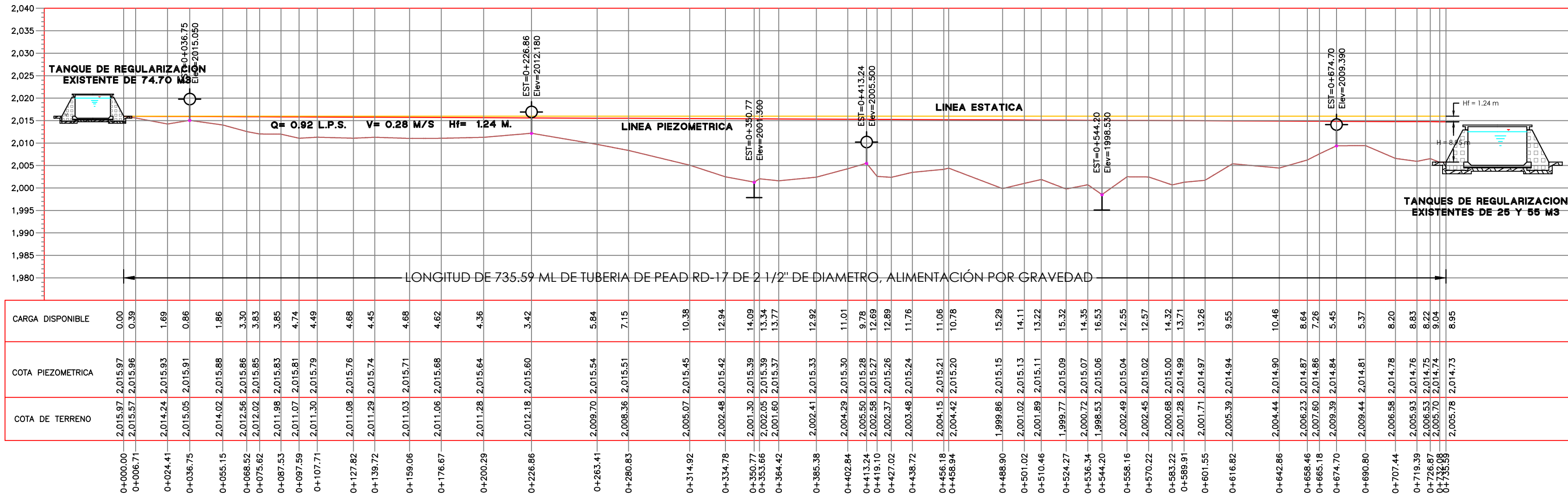
PERFIL LINEA DE ALIMENTACION ESCALA HORIZONTAL 1 : 2000 ESCALA VERTICAL 1 : 800
