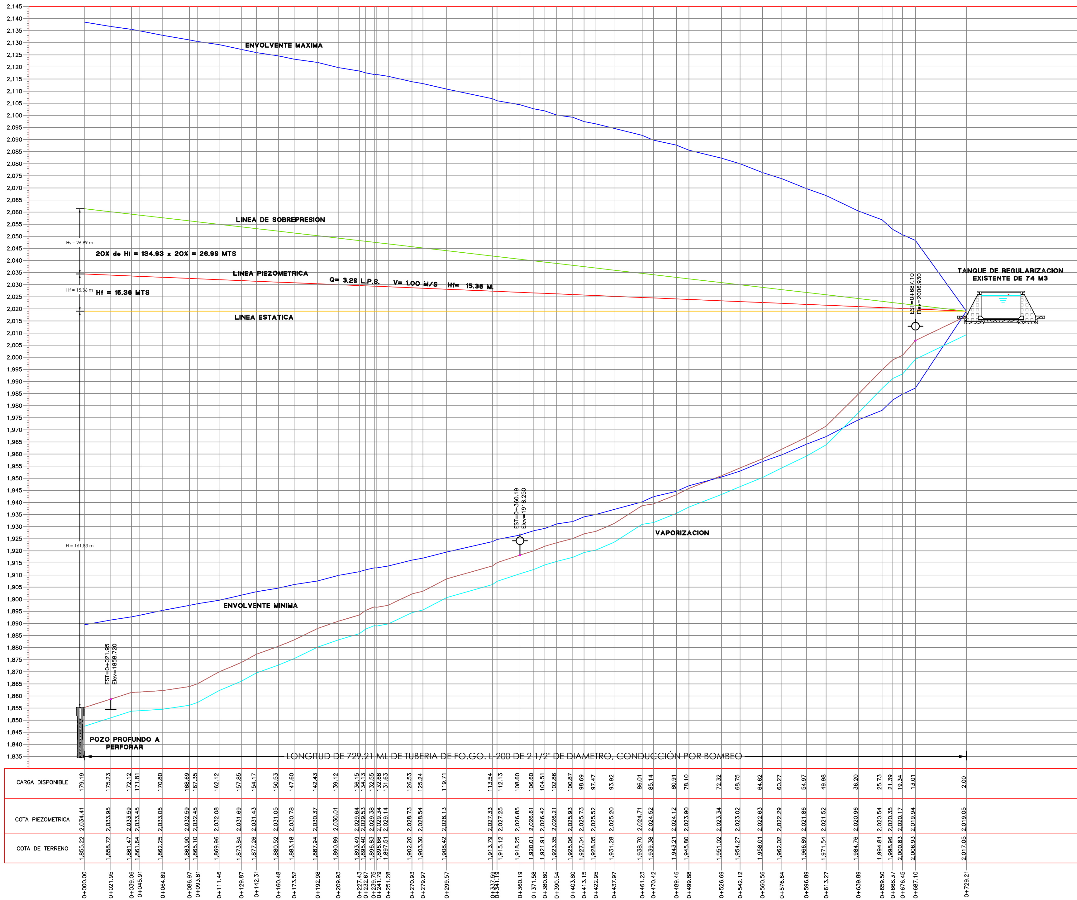
PERFIL LINEA DE CONDUCCION ESCALA HORIZONTAL 1 : 2000 ESCALA VERTICAL 1 : 1000
