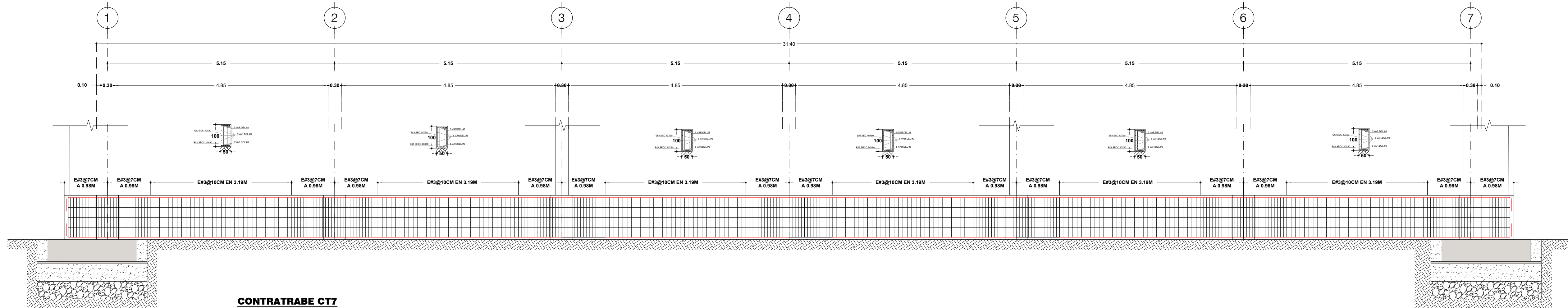
CONTRATRABE CT7
