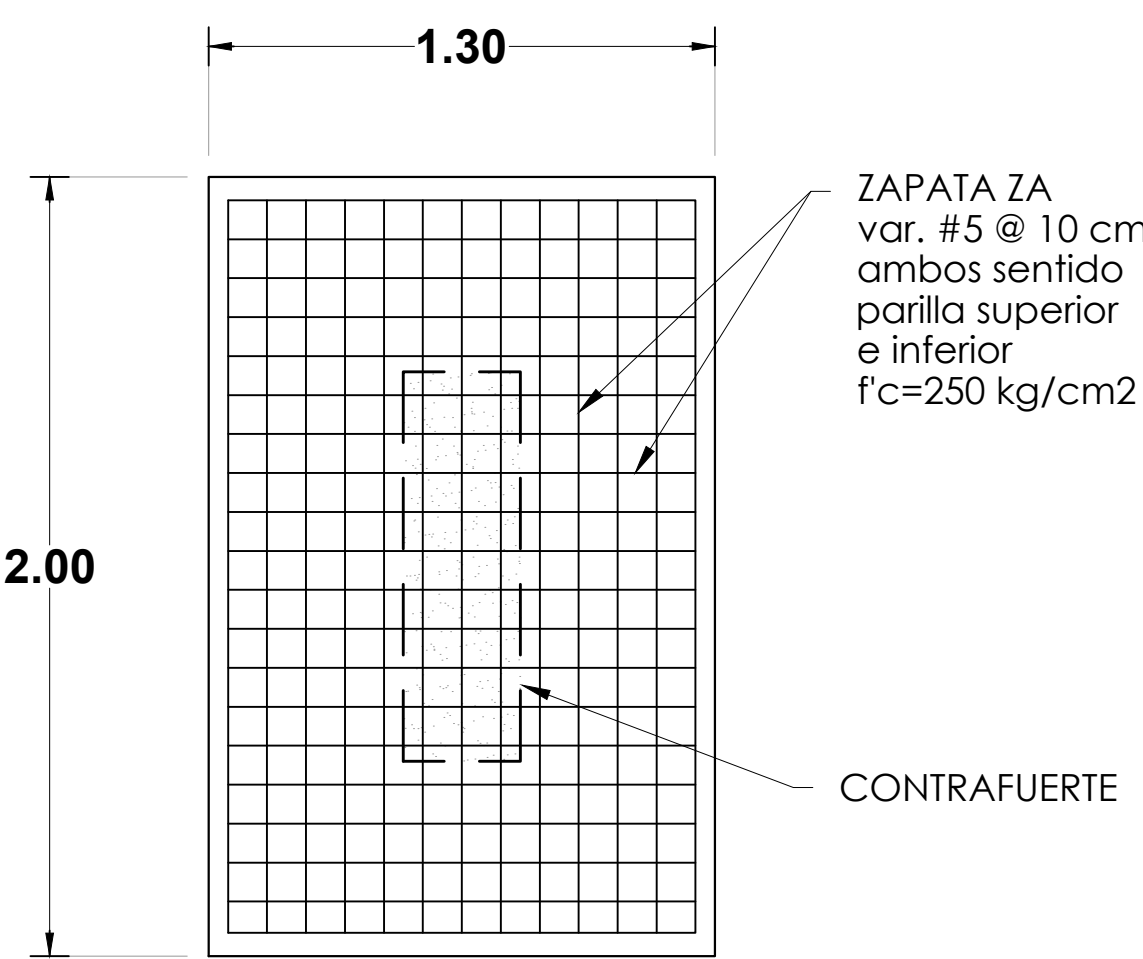
PLANTA ZA ESC. S/E
