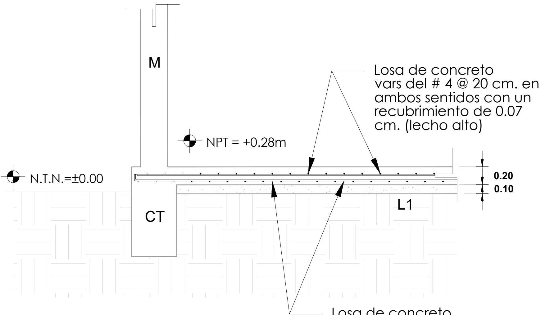
CORTE LOSA INFERIOR ESC. S/E
