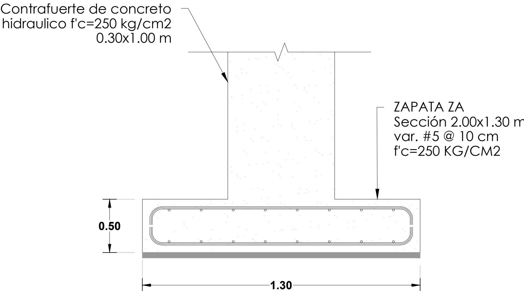
CORTE ZA ESC. S/E
