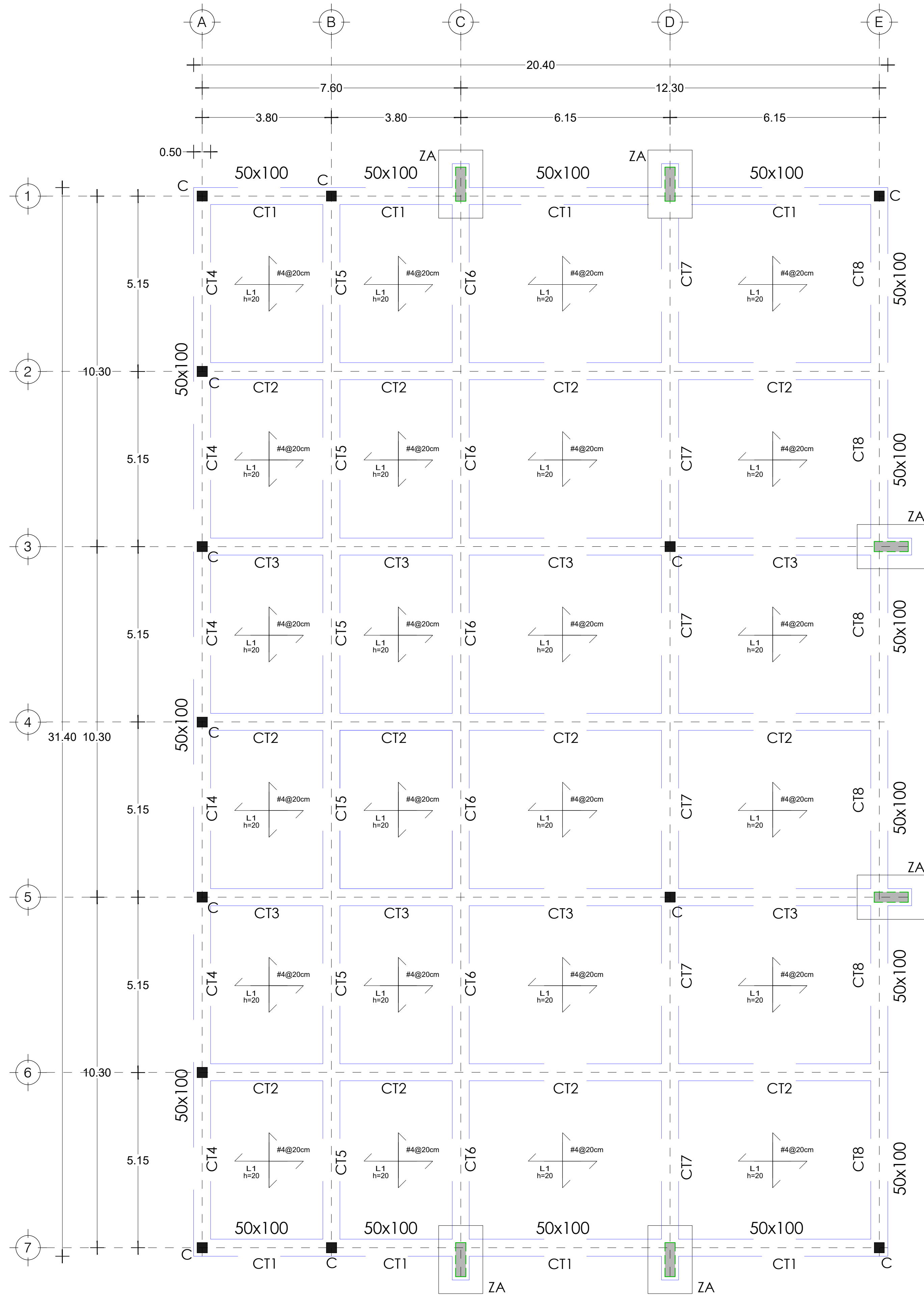
PLANTA DE CIMENTACIÓN CAMARA DE AIREACIÓN ESCALA: 1:75
