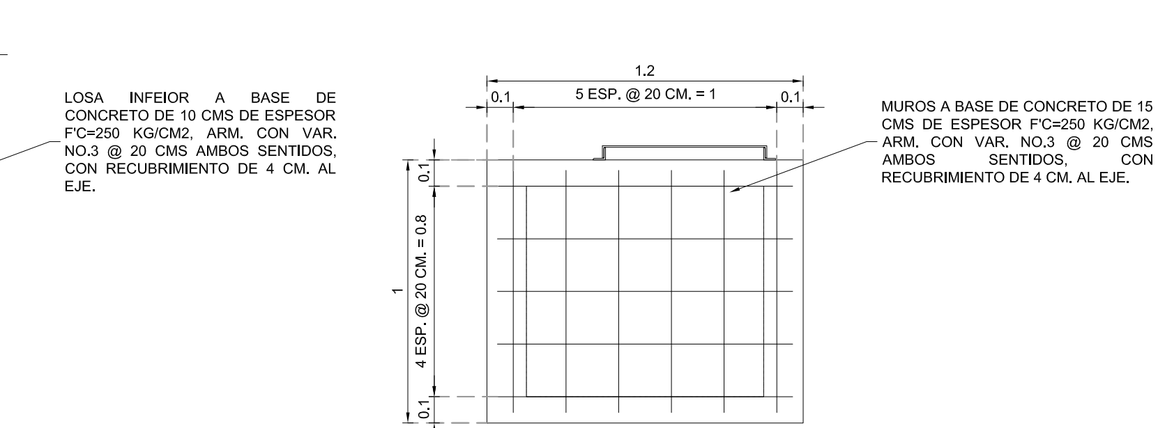
ELEVACIÓN. ARMADO EN MUROS. ESCALA 1:10
