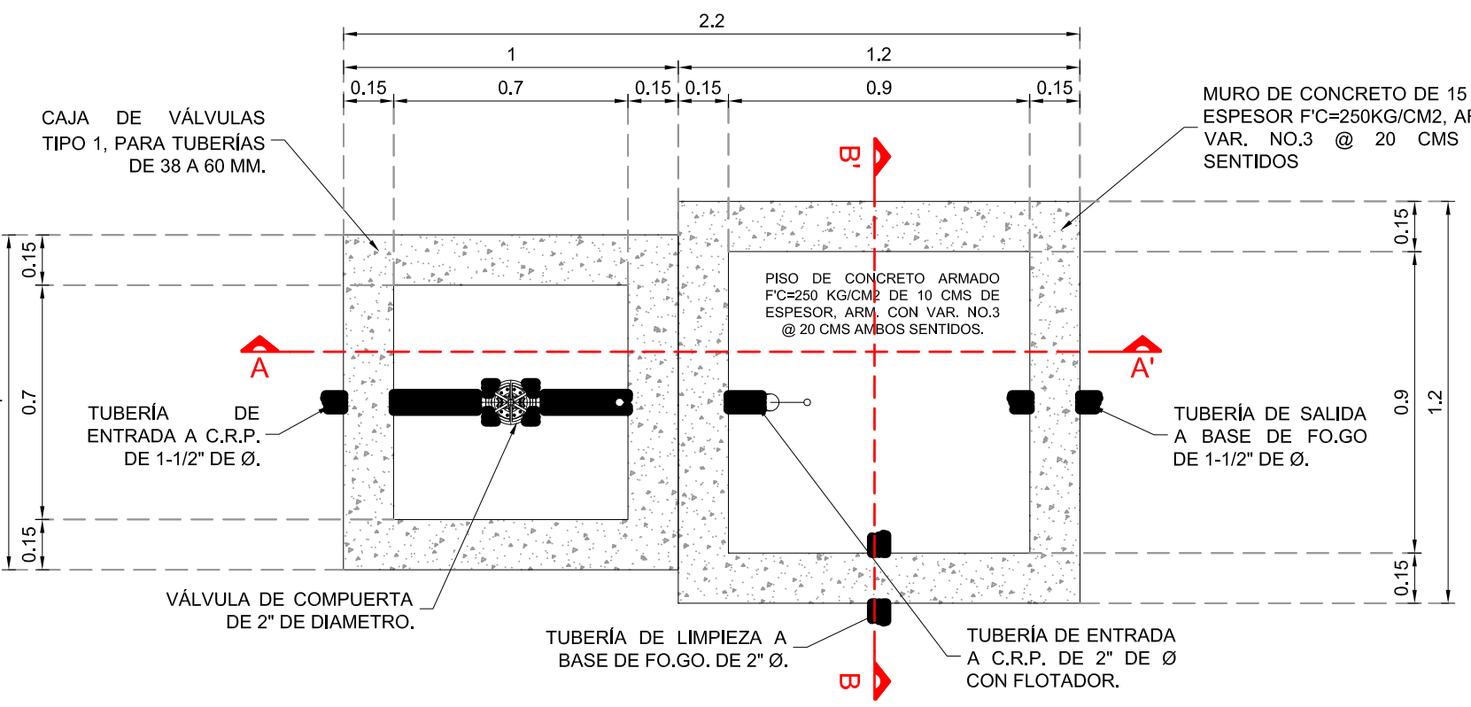
PLANTA GENERAL. CAJA ROMPEDORA DE PRESIÓN. ESCALA 1:10
