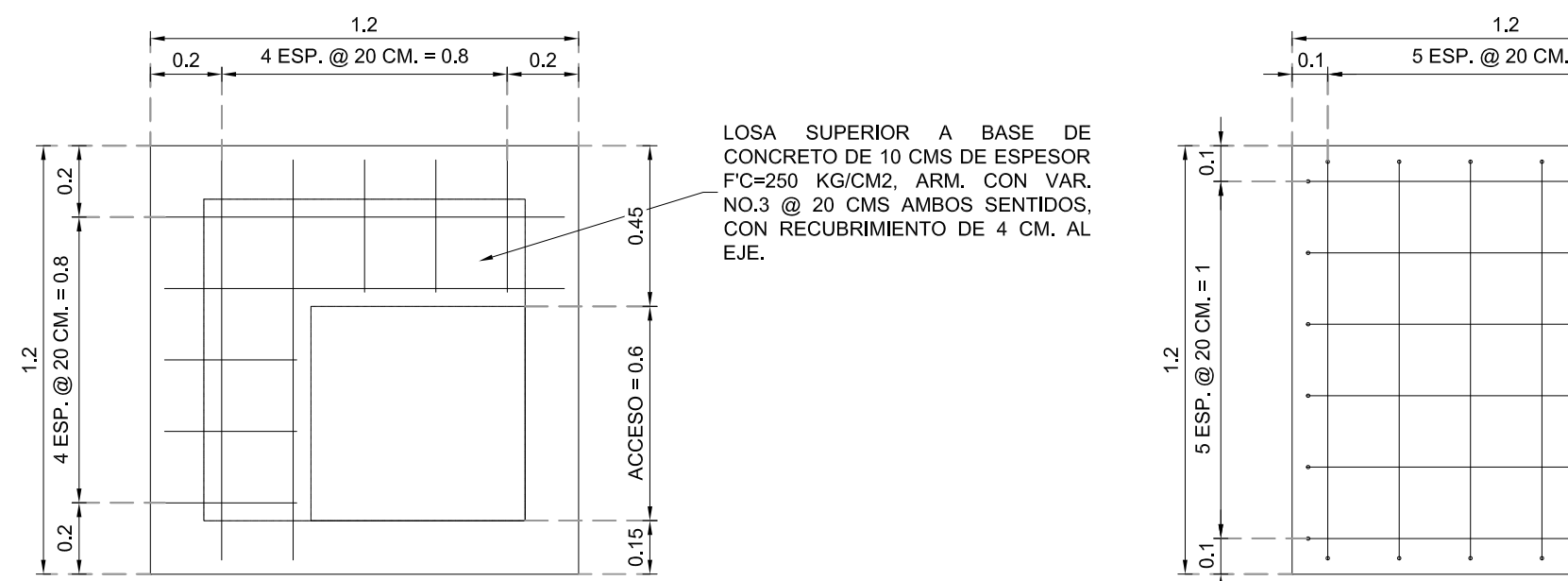
PLANTA GENERAL. LOSA SUPERIOR. ESCALA 1:10
