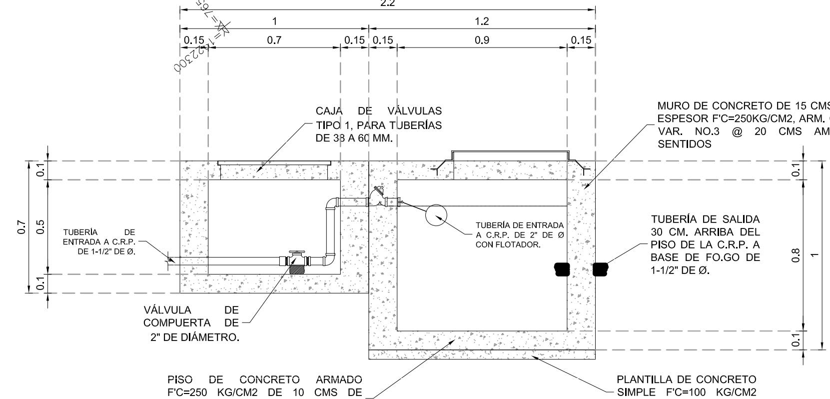
ELEVACIÓN CORTE A-A'. CAJA ROMPEDORA DE PRESIÓN. ESCALA 1:10
