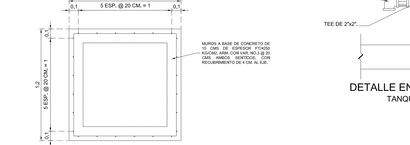
PLANTA. MUROS DE CONCRETO ARMADO. ESCALA 1:10
