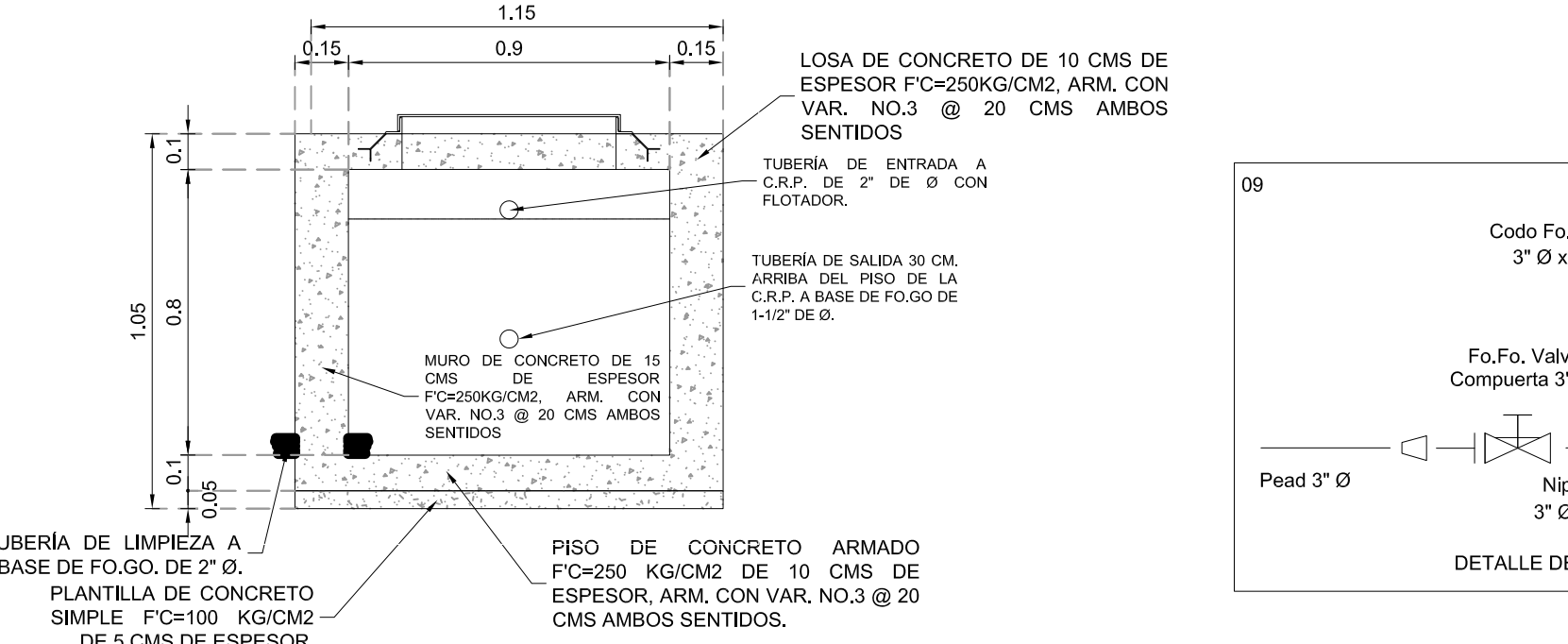
ELEVACIÓN CORTE B-B'. CAJA ROMPEDORA DE PRESIÓN. ESCALA 1:10
