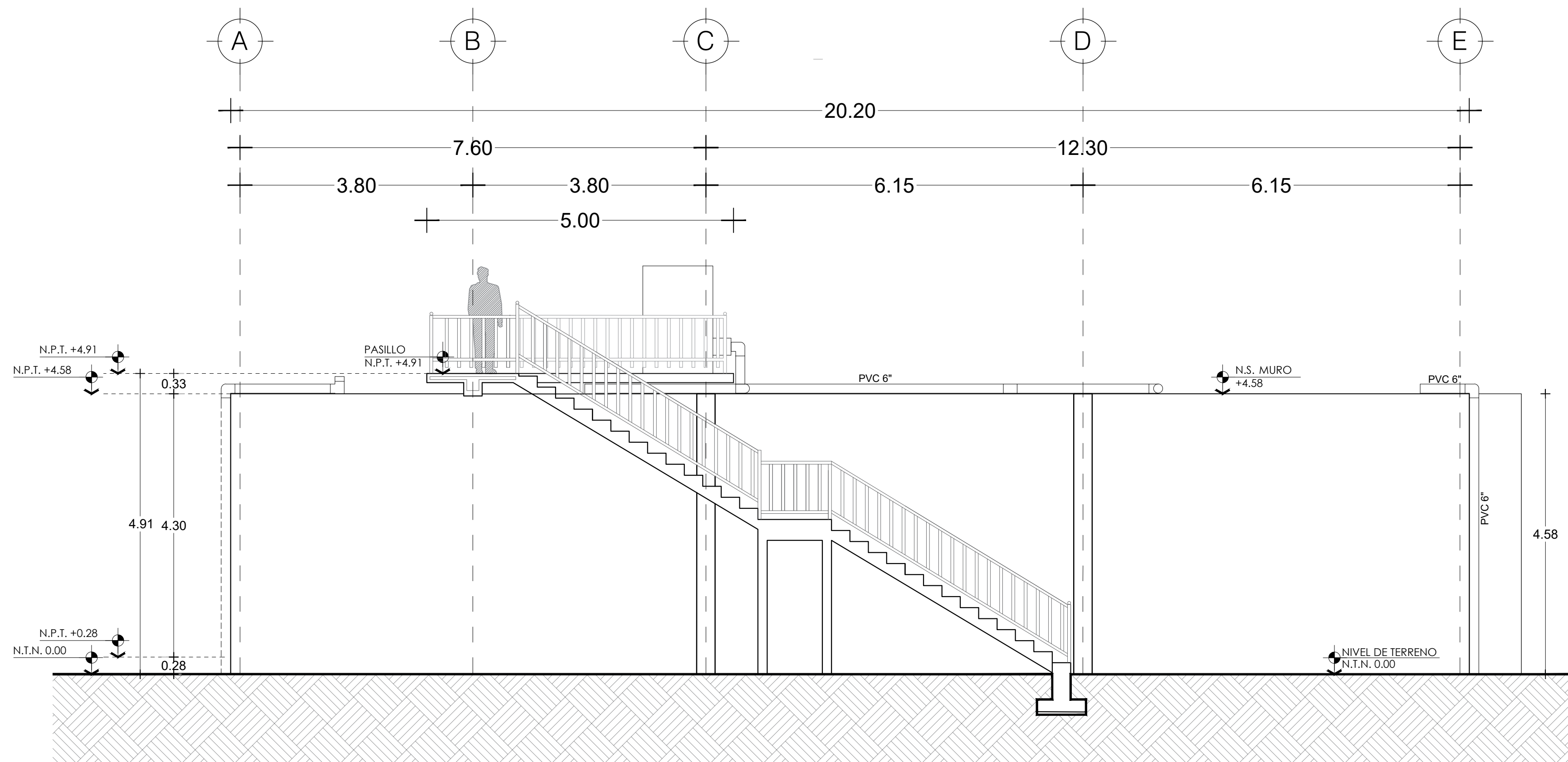
ALZADO CÁMARA DE AIREACIÓN
