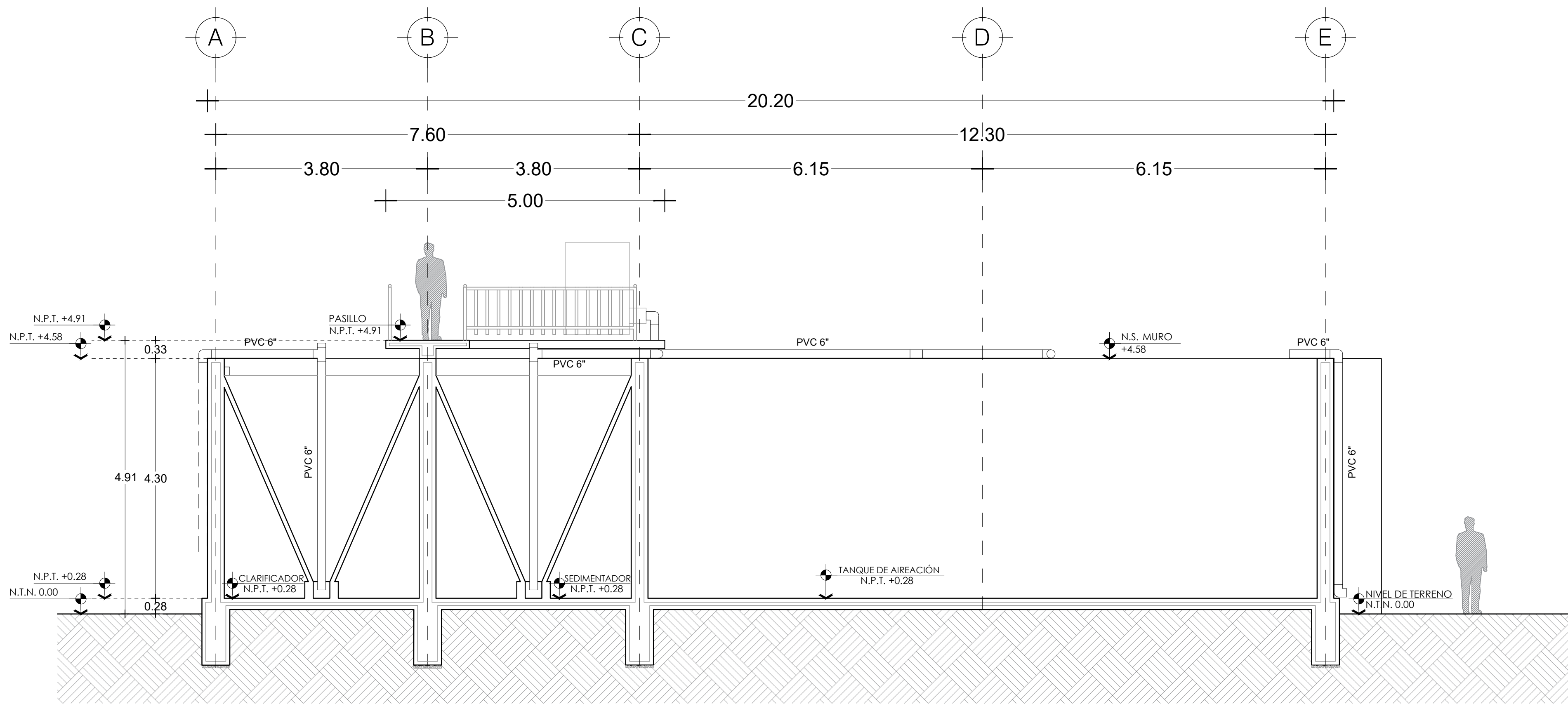
CORTE A-A' CÁMARA DE AIREACIÓN
