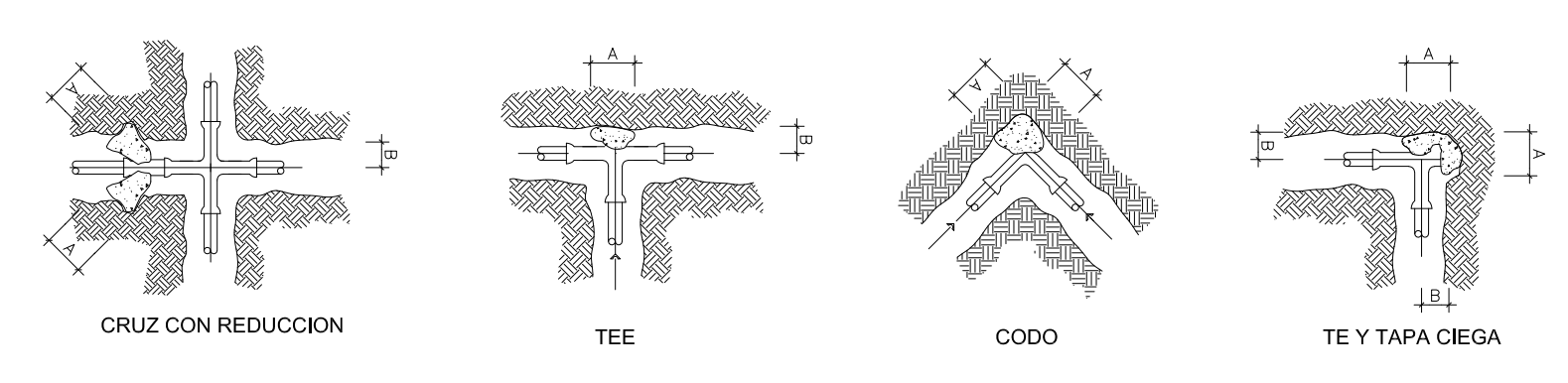
ATRAQUES PARA PIEZAS ESPECIALES. PLANTA GENERAL. SIN ESCALA
