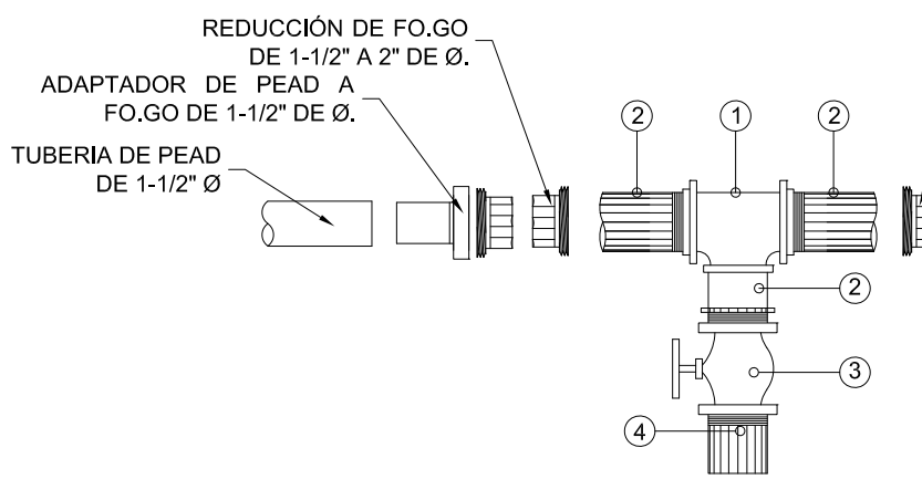
DETALLE VÁLVULA DE DESFOQUE. SIN ESCALA
