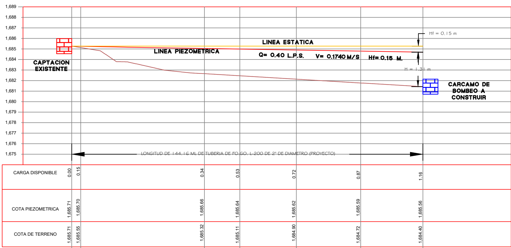
PERFIL LINEA DE CONDUCCION POR GRAVEDAD ESCALA HORIZONTAL 1 : 1000 ESCALA VERTICAL 1 : 200
