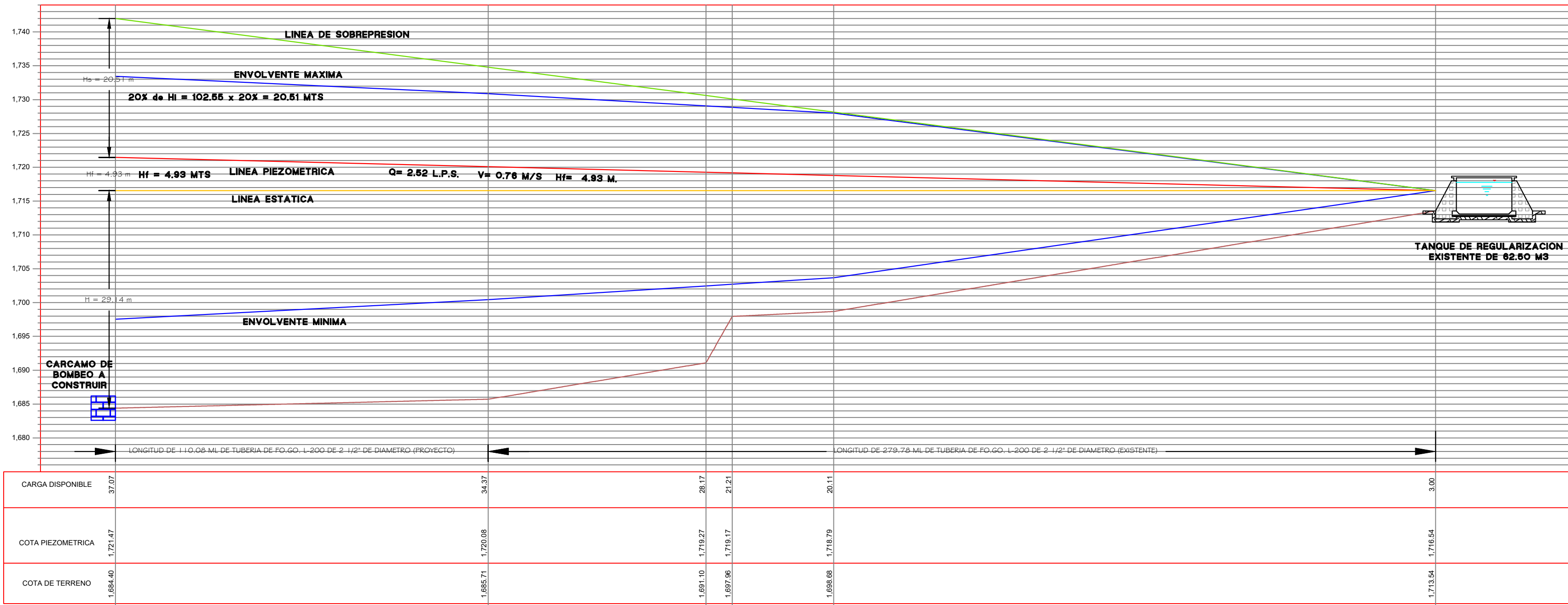
PERFIL LINEA DE CONDUCCION POR BOMBEO SECTOR 2 ESCALA HORIZONTAL 1 : 1000 ESCALA VERTICAL 1 : 500
