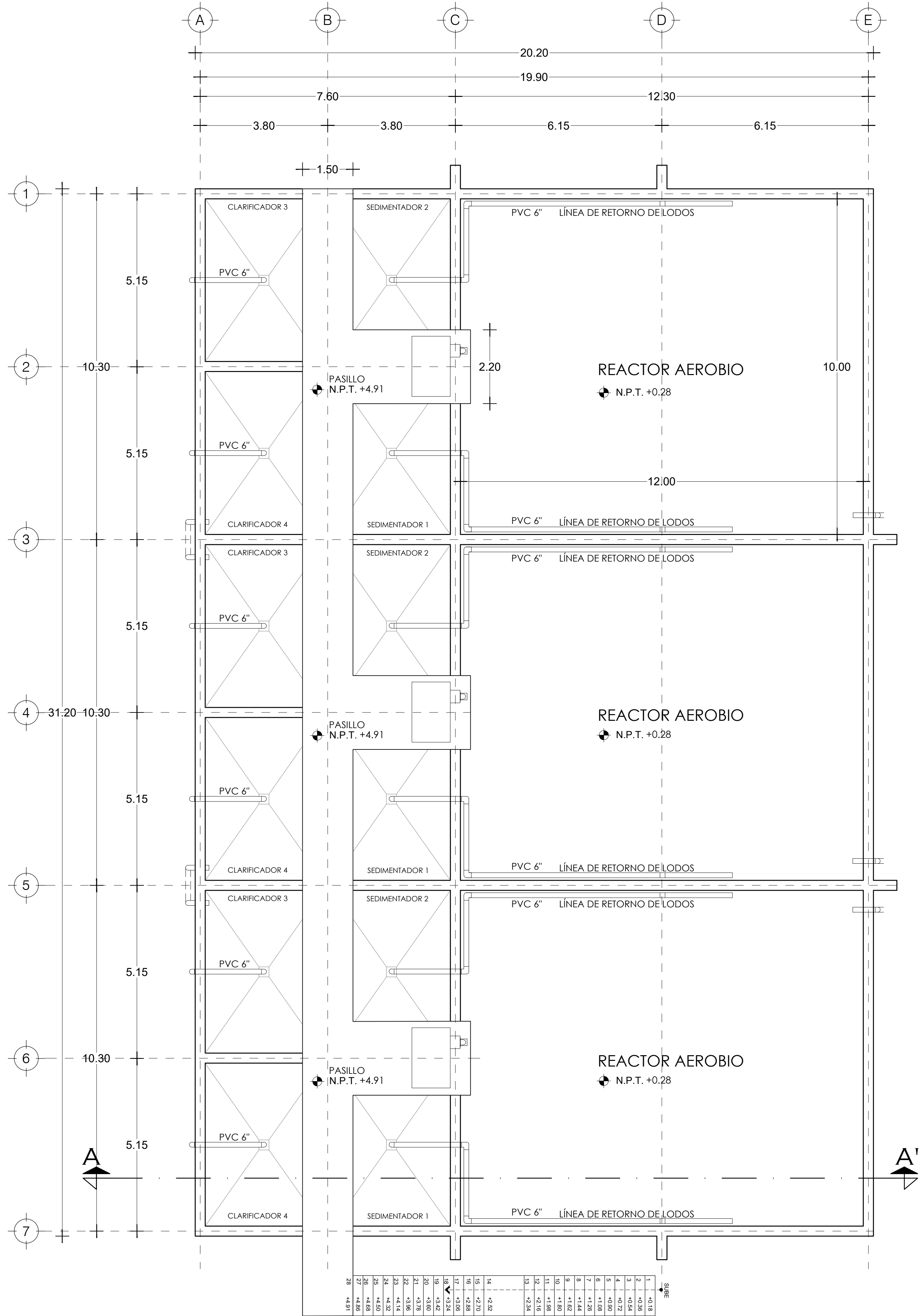
PLANTA ARQUITECTONICA CÁMARA AIREACIÓN ESC. 1:75
