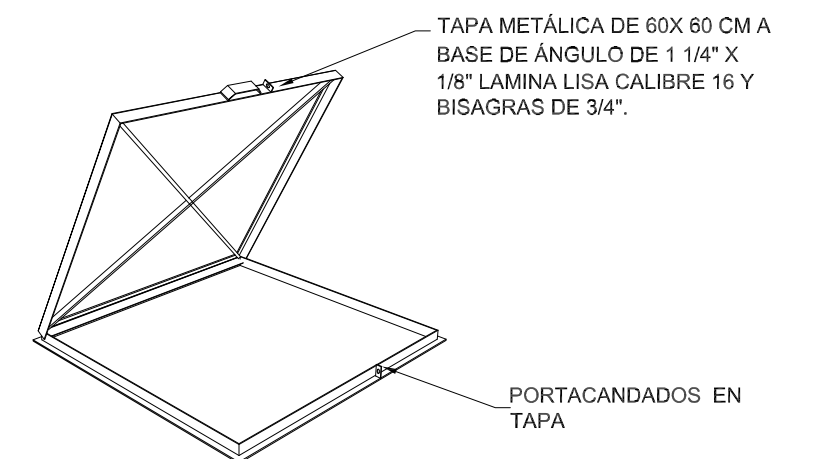
DETALLE EN TAPA. TAPA METÁLICA EN CAJA DE CAPTACIÓN. SIN ESCALA.
