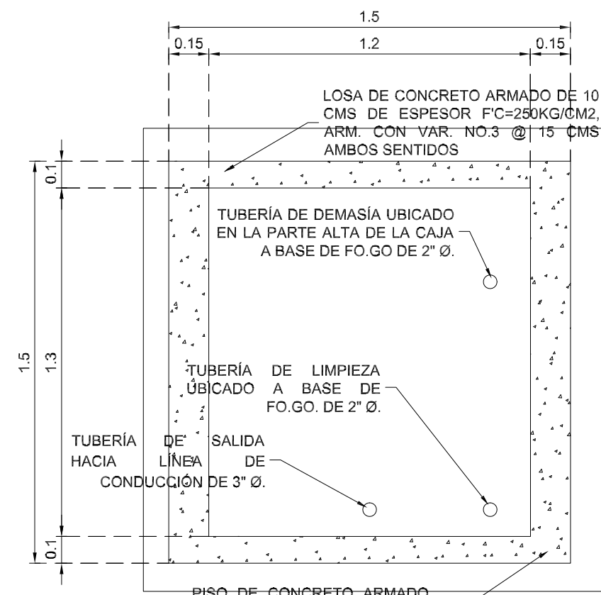
ELEVACIÓN CORTE A-A'. CAJA DE CAPTACIÓN. ESCALA 1:10
