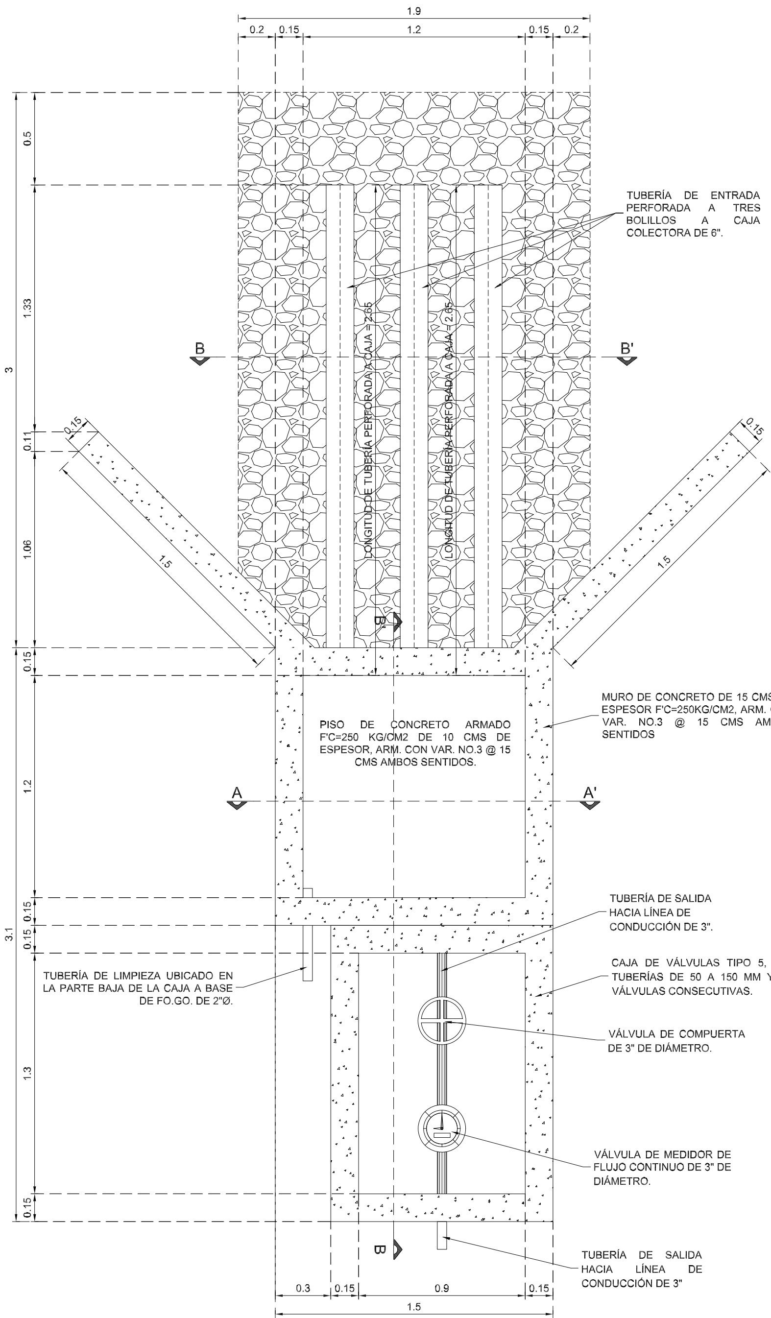
PLANTA GENERAL. CAJA DE CAPTACIÓN. ESCALA 1:10
