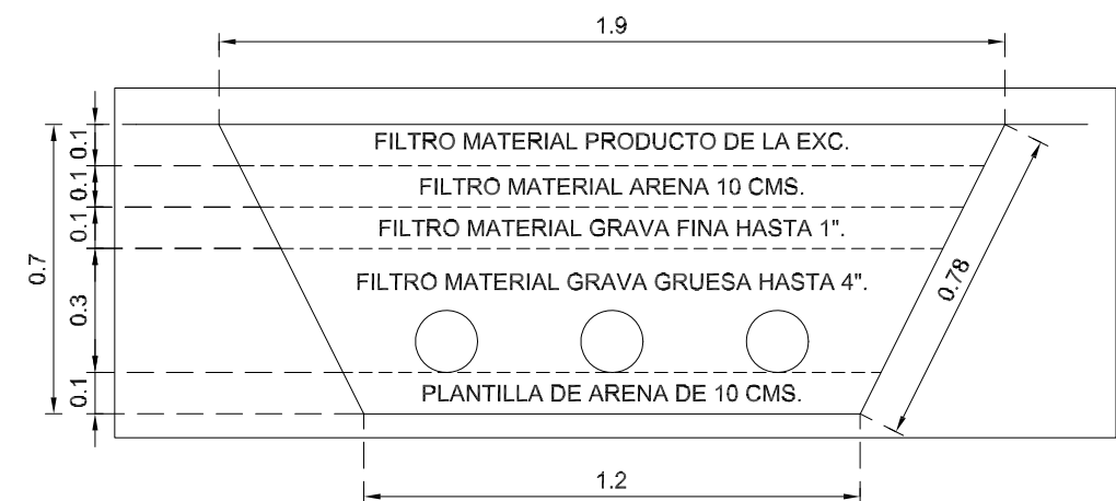
ELEVACIÓN CORTE B-B'. CAJA DE CAPTACIÓN. ESCALA 1:10
