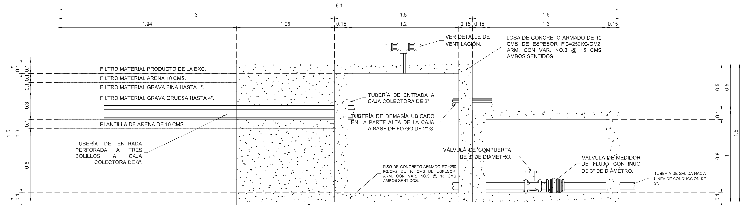
ELEVACIÓN CORTE B-B'. CAJA DE CAPTACIÓN. ESCALA 1:10
