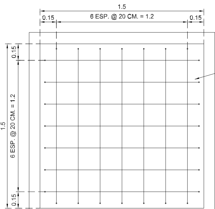
PLANTA GENERAL. LOSA INFERIOR. ESCALA 1:10
