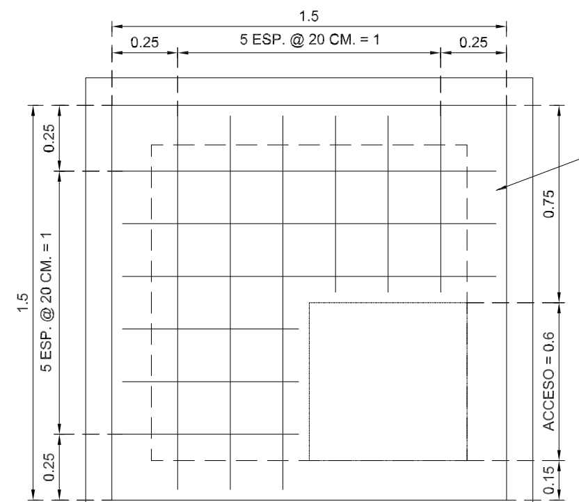
PLANTA GENERAL. LOSA SUPERIOR. ESCALA 1:10
