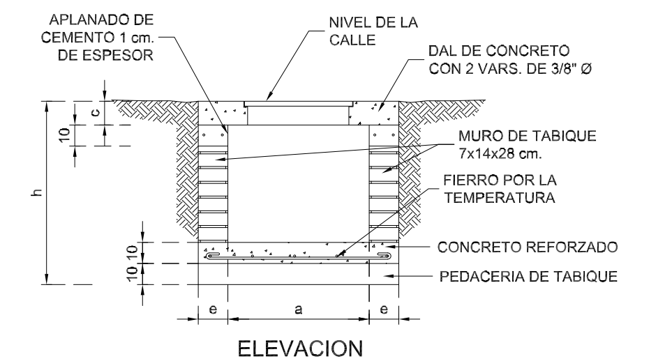
ELEVACION
