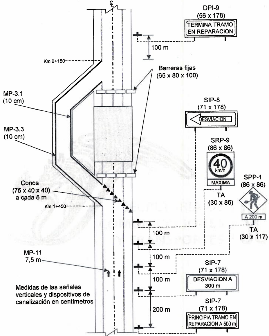
FIGURA 1.- Ejemplo de representación del señalamiento para protección en obras
