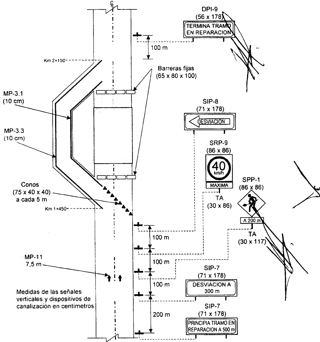
FIGURA 1.- Ejemplo de representación del señalamiento para protección en obras
