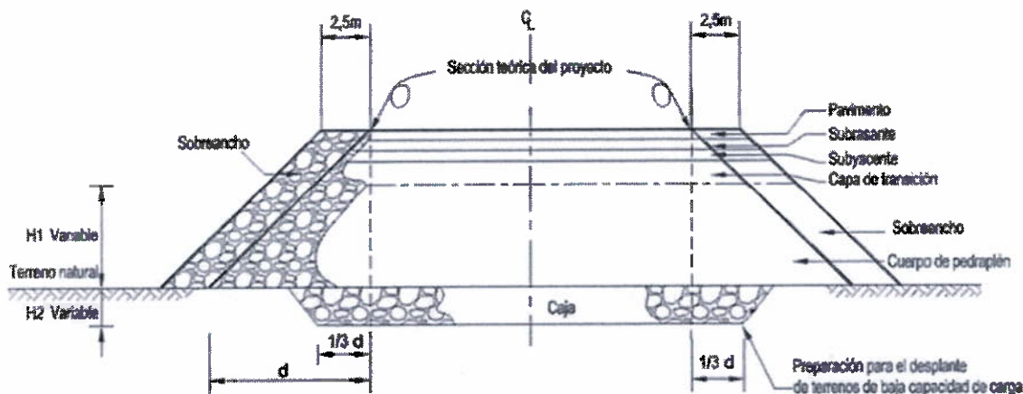
FIGURA 2.- Sección transversal
