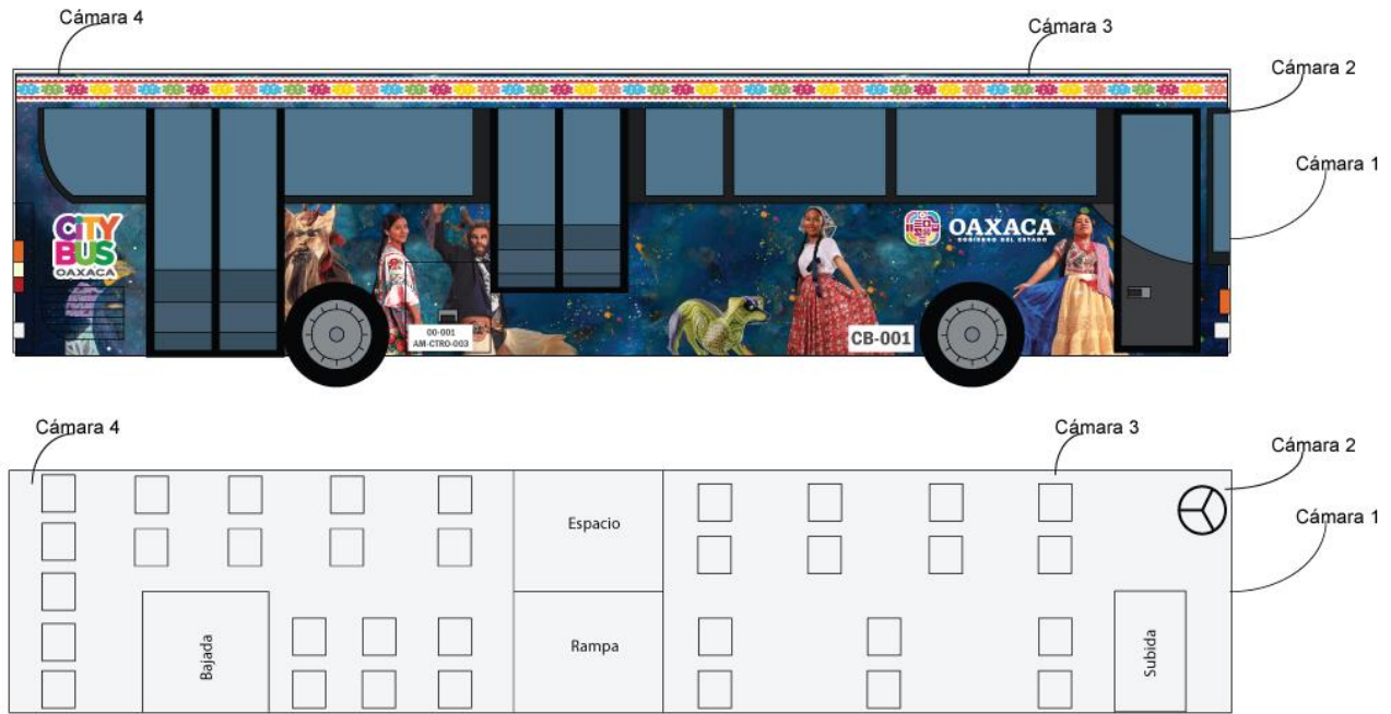
FIGURA 1.- DISTRIBUCIÓN DE CÁRAMAS PARA VIDEOVIGILANCIA
