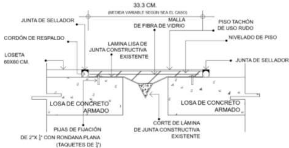
DIAGRAMA DE REPARACIÓN Y MANTENIMIENTO DE JUNTAS CONSTRUCTIVAS EN LOS EDIFICIOS DEL 1 AL 8
