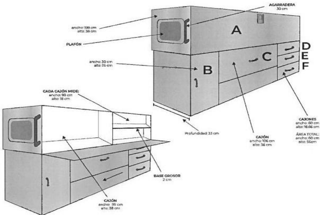
CAJA DE HERRAMIENTA LATERAL DEL COSTADO IZQUIERDO:
