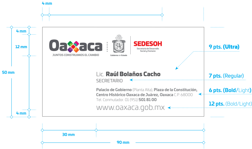
Tarjeta de presentación (Anotaciones en milímetros)
