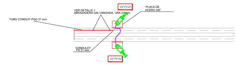
SOPORTE P/ INSTALACIÓN DE PLANTA DE MONTAJE DE CÁMARAS
