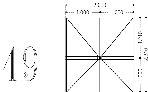
Puerta de emergencia espectadores (P-E1) 1 pza
