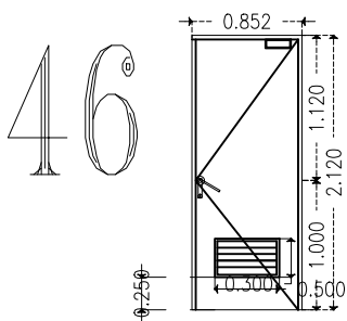
Baños mujeres con rejilla y cierra puertas. (P-1) 1 pza
