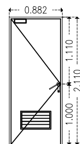
Baños hombres con rejilla y cierra puertas. (P-2) 1 pza
