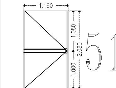
Puerta de emergencia espectadores (P-E3) 1 pza
